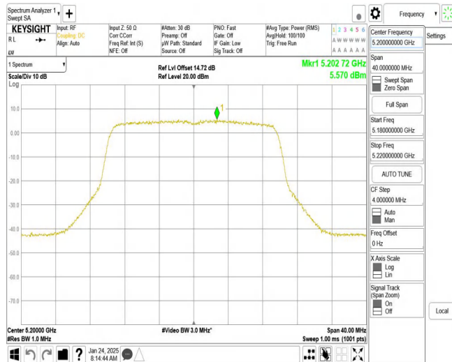
11AX20MIMO_Ant1_5200
