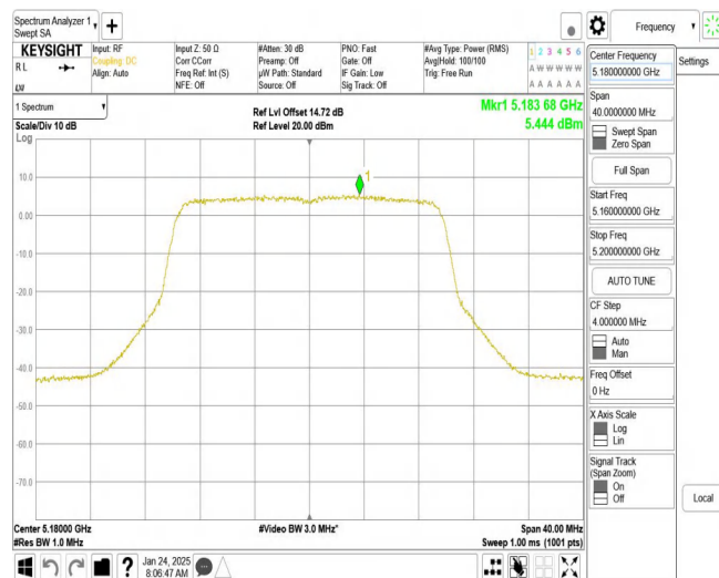
11AX20MIMO_Ant1_5180
