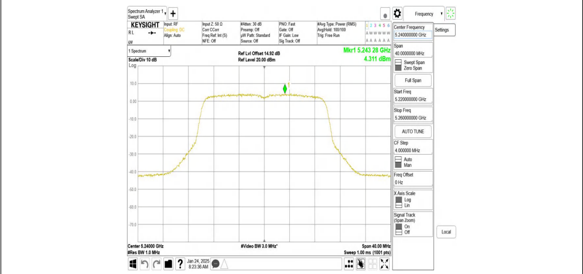
11AX20MIMO_Ant2_5240
