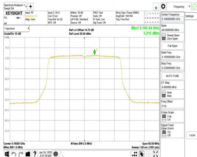
11AX40MIMO_Ant1_5190
