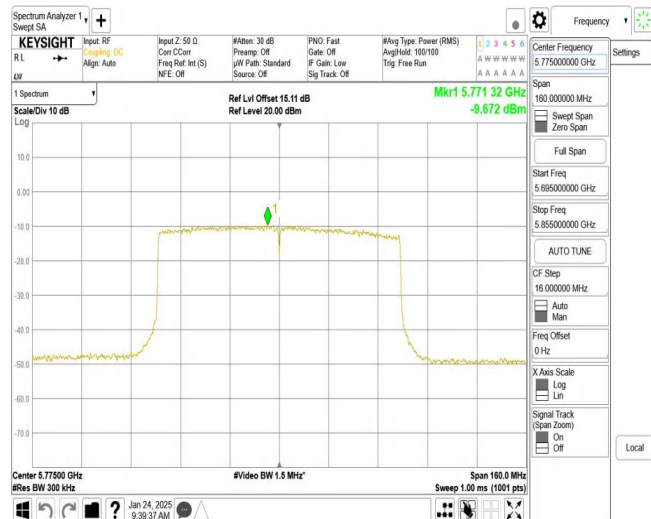
11AX80MIMO_Ant1_5775
