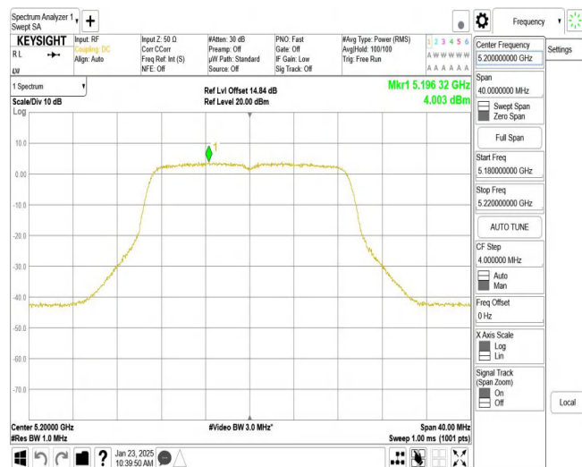
11AC20MIMO_Ant2_5200
