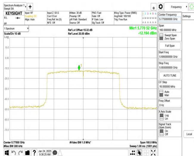
11AX80MIMO_Ant2_5775
