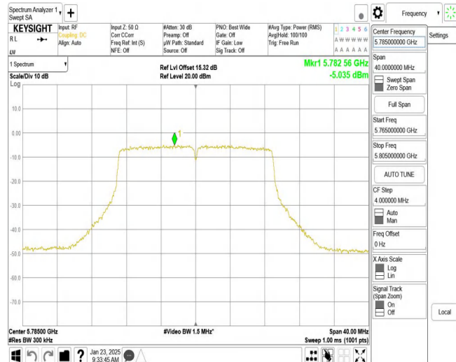
11N20MIMO_Ant2_5785
