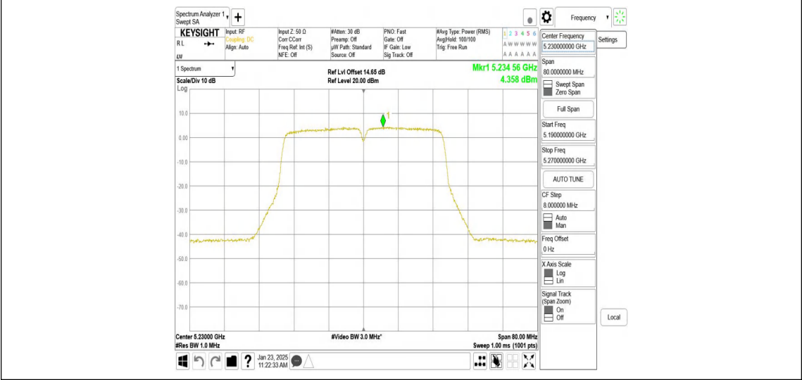
11AC40MIMO_Ant1_5230
