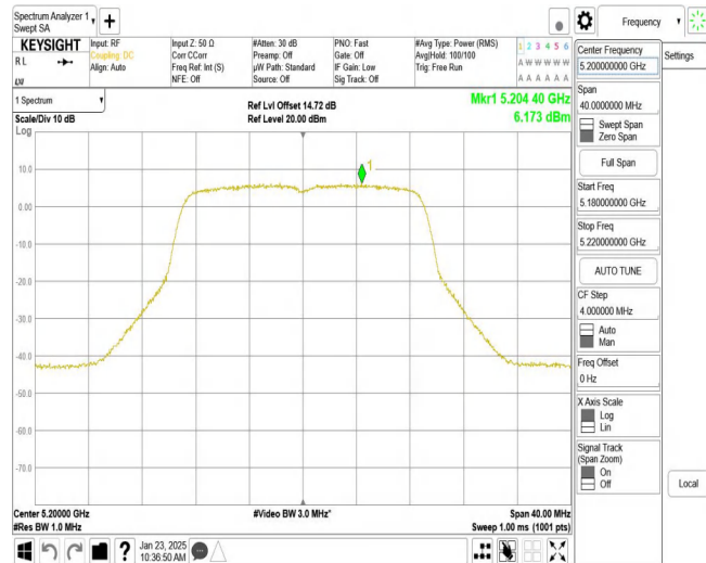
11AC20MIMO_Ant1_5200
