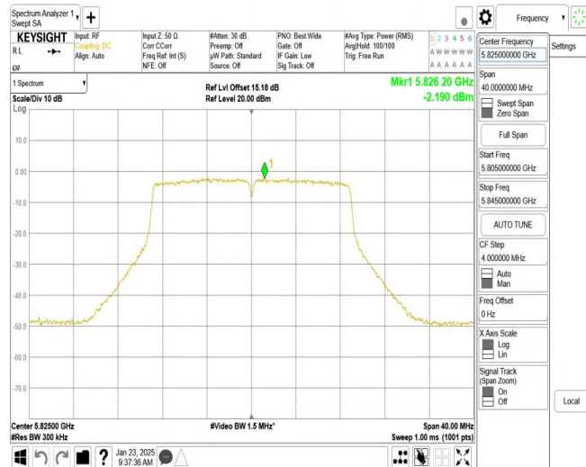
11N20MIMO_Ant1_5825
