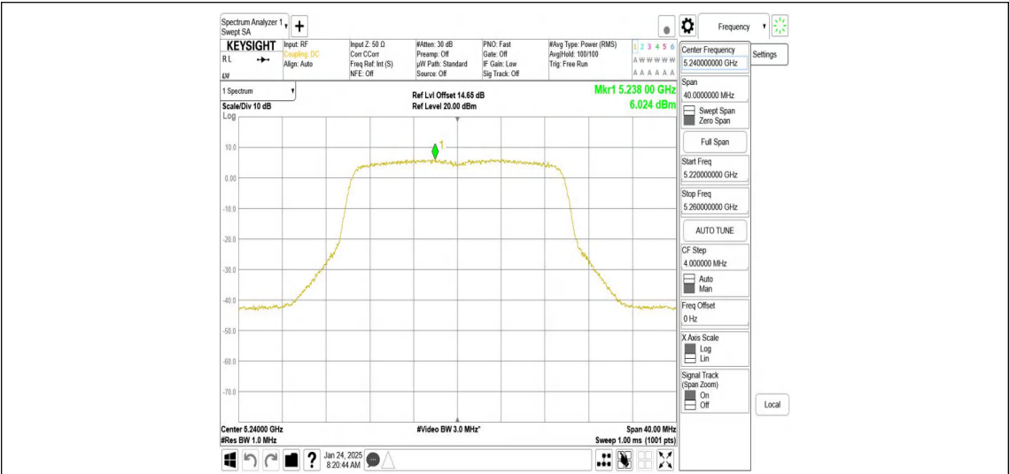
11AX20MIMO_Ant1_5240
