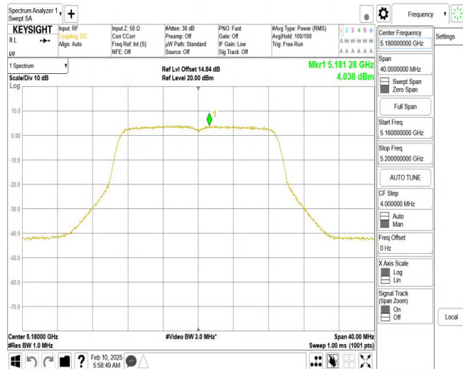
11AC20MIMO_Ant2_5180
