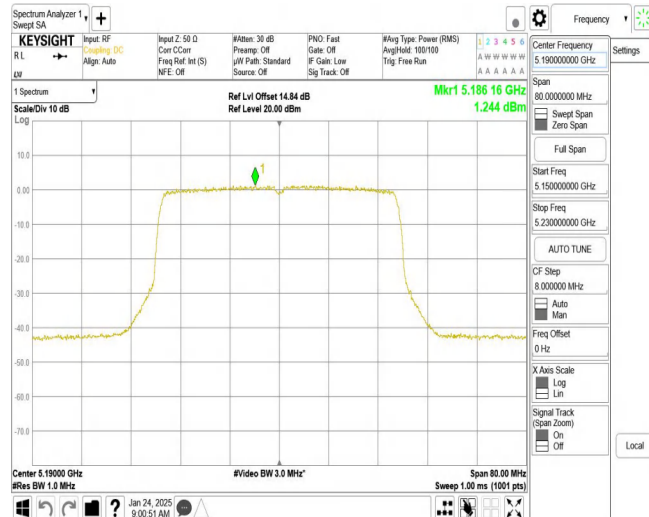
11AX40MIMO_Ant2_5190
