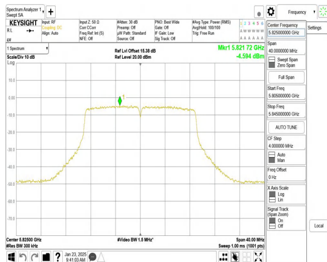
11N20MIMO_Ant2_5825
