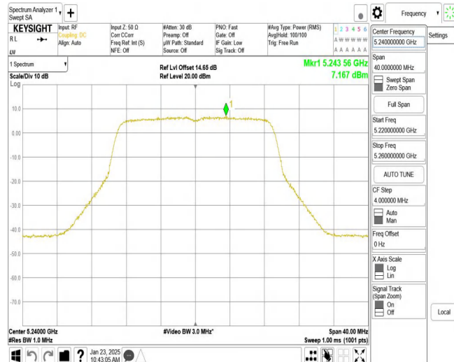
11AC20MIMO_Ant1_5240
