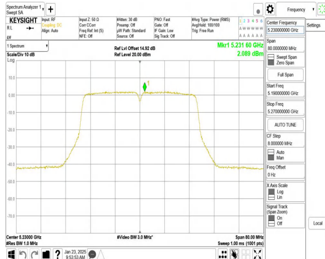
11N40MIMO_Ant2_5230
