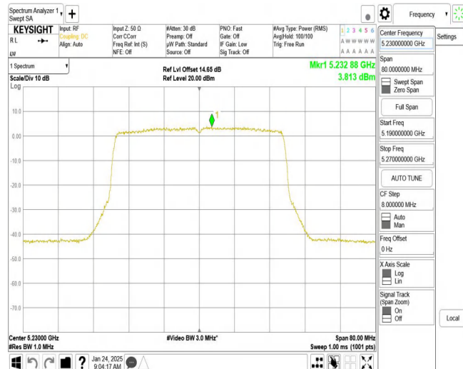
11AX40MIMO_Ant1_5230
