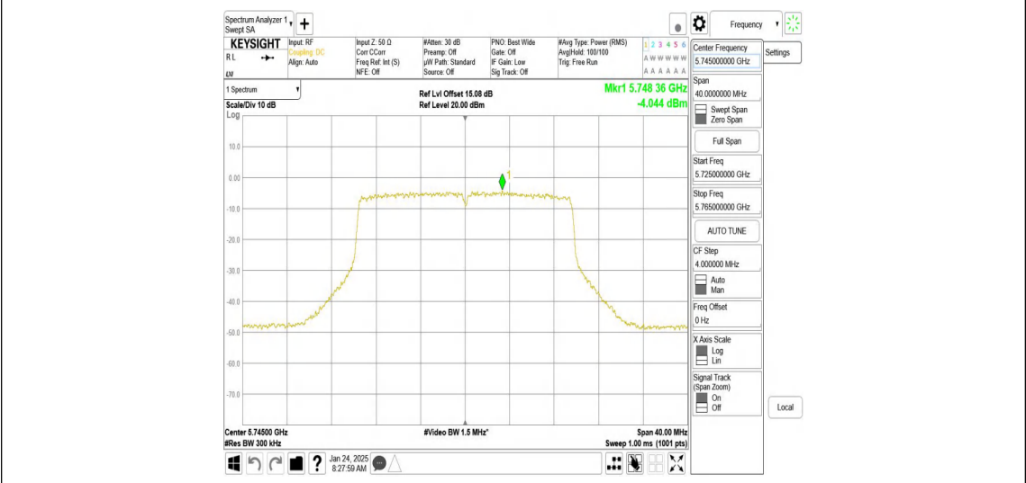
11AX20MIMO_Ant1_5745
