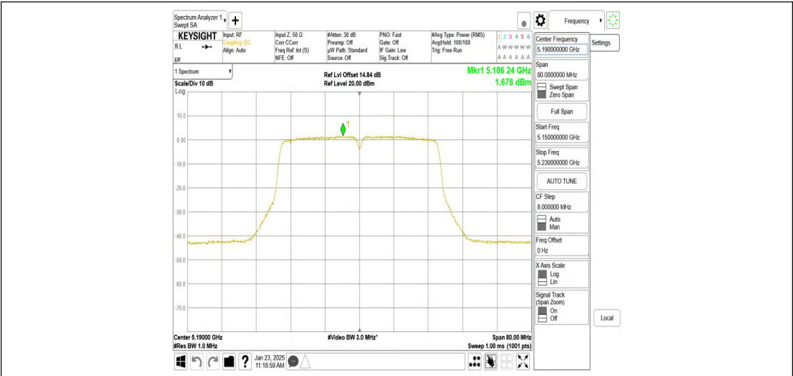
11AC40MIMO_Ant2_5190
