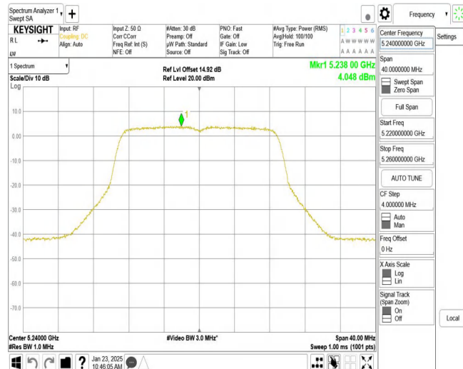
11AC20MIMO_Ant2_5240
