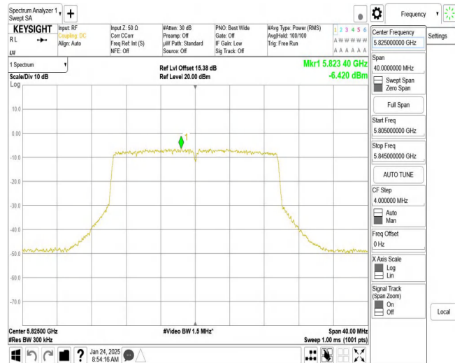
11AX20MIMO_Ant2_5825
