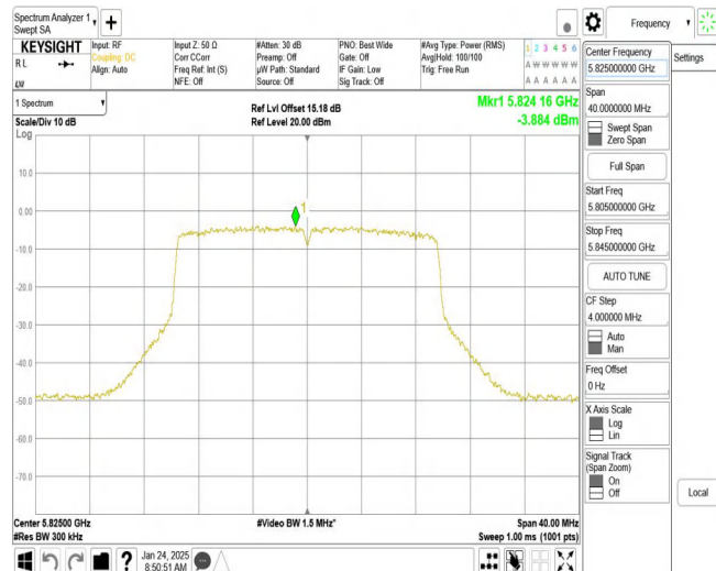
11AX20MIMO_Ant1_5825
