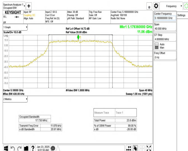
11N20MIMO_Ant1_5180
