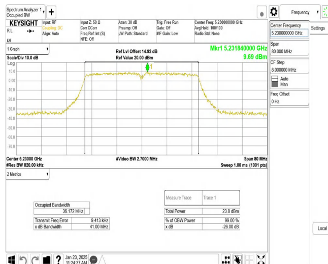
11AC40MIMO_Ant2_5230
