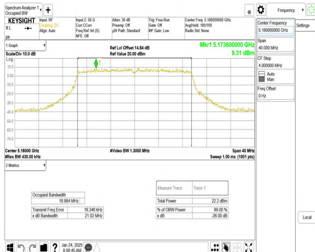
11AX20MIMO_Ant2_5180
