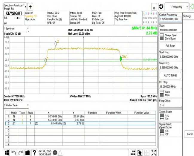
11AX80MIMO_Ant2_5775
