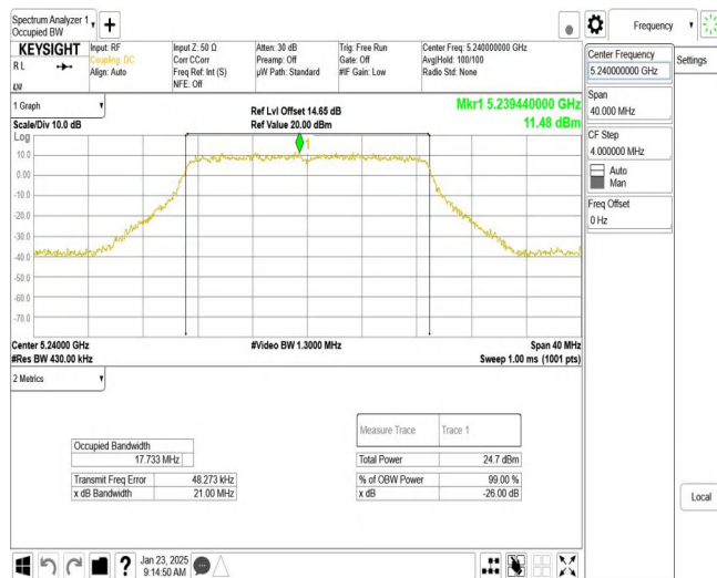
11N20MIMO_Ant1_5240
