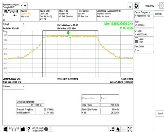
11AC20MIMO_Ant1_5200
