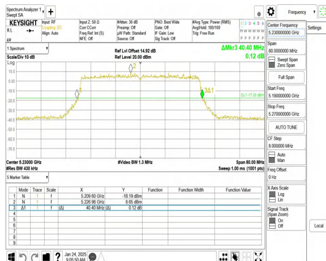
11AX40MIMO_Ant2_5230
