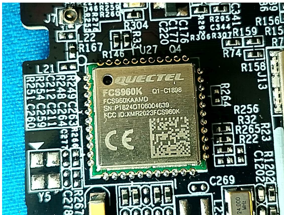
Bluetooth&Wifi Module
