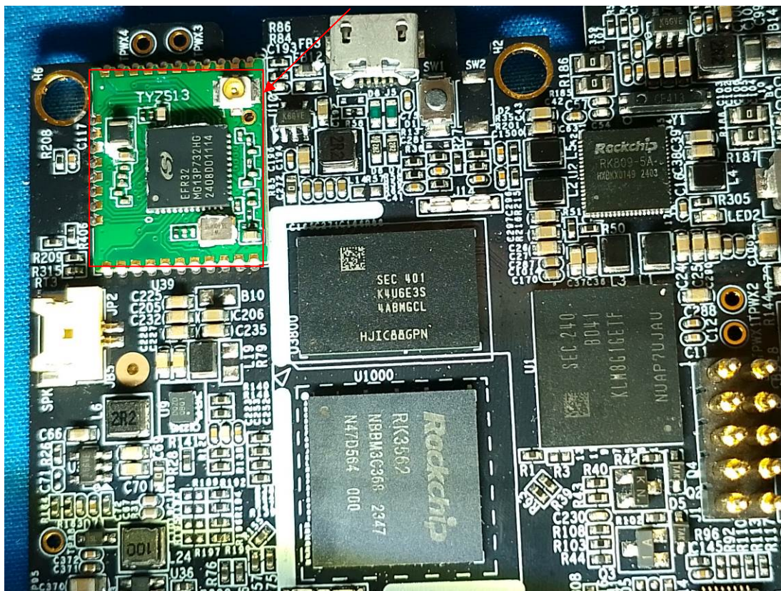
ZigBee Module
