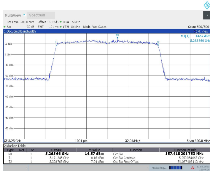
11AX160MIMO_Ant9_5250
