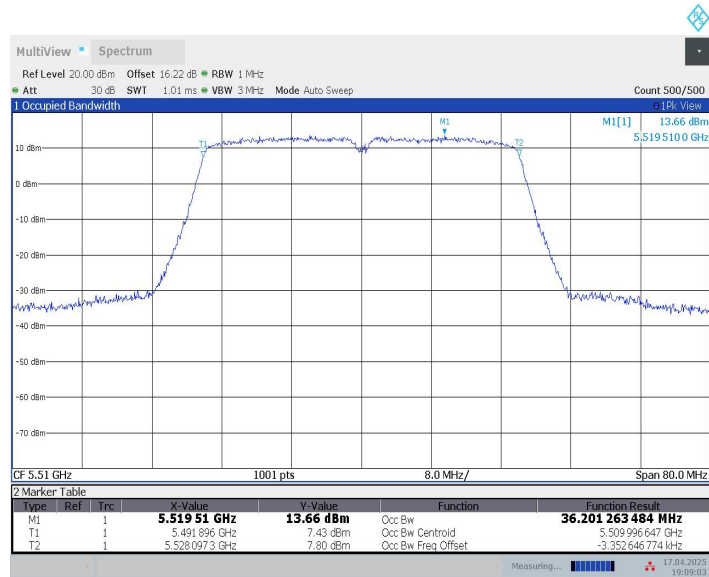
11N40MIMO_Ant9_5510
