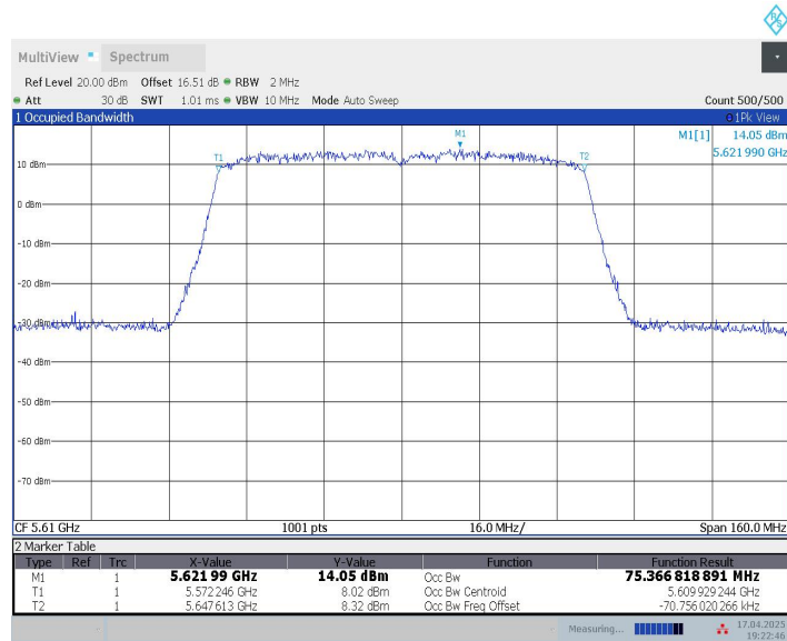
11AC80MIMO_Ant9_5610
