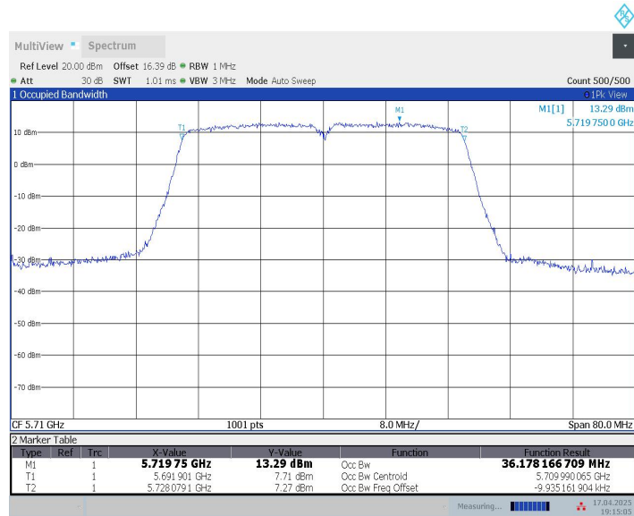
11N40MIMO_Ant9_5710
