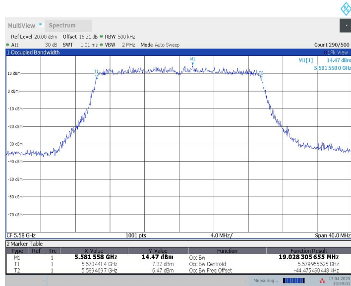
11AX20MIMO_Ant9_5580
