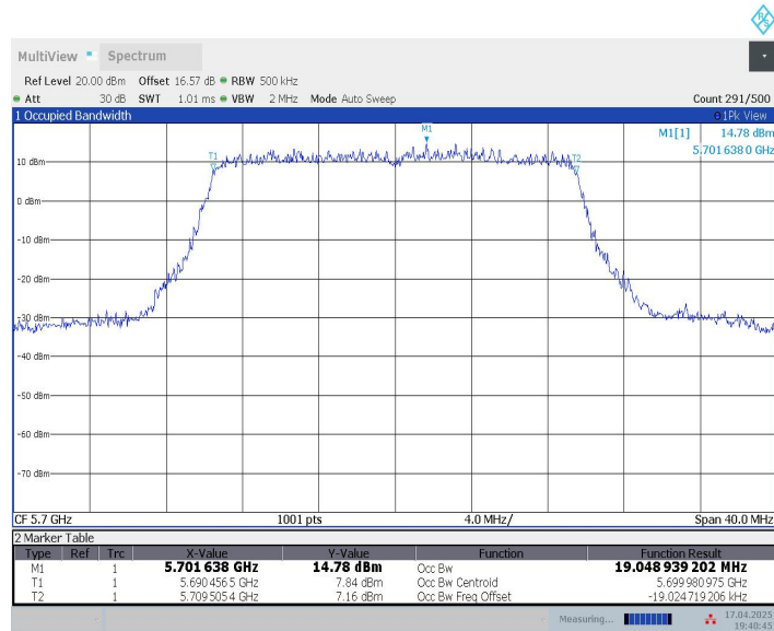
11AX20MIMO_Ant9_5700
