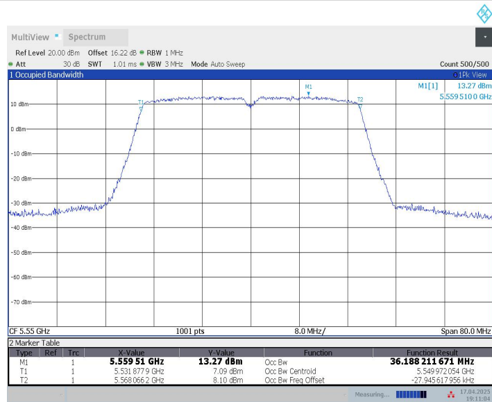
11N40MIMO_Ant9_5550
