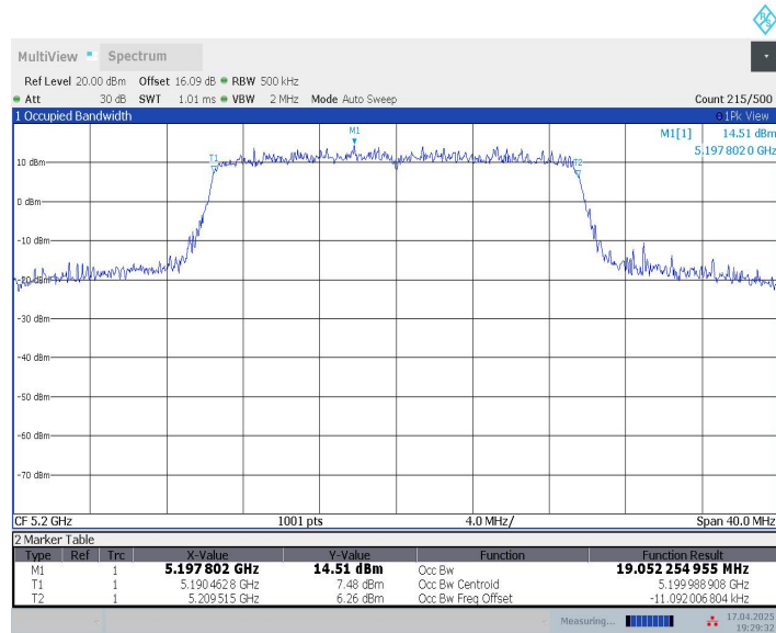
11AX20MIMO_Ant9_5200
