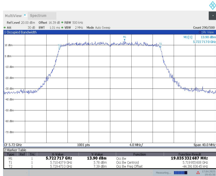
11AX20MIMO_Ant9_5720
