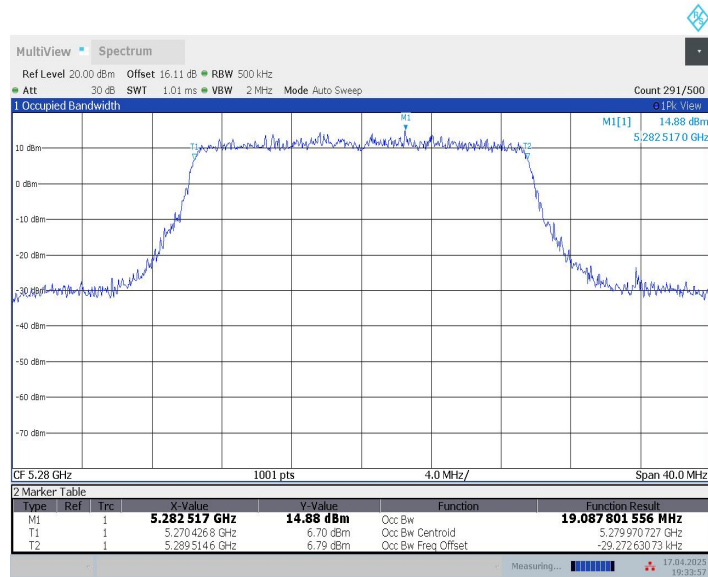
11AX20MIMO_Ant9_5280
