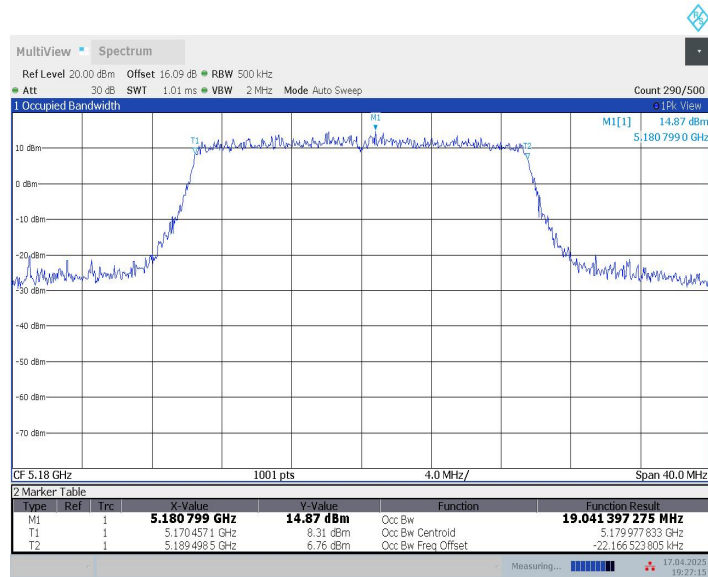
11AX20MIMO_Ant9_5180
