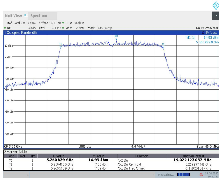
11AX20MIMO_Ant9_5260
