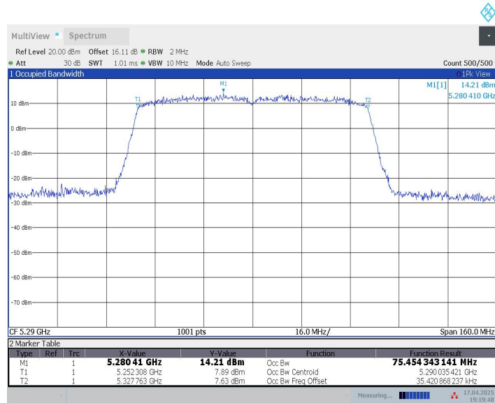
11AC80MIMO_Ant9_5290
