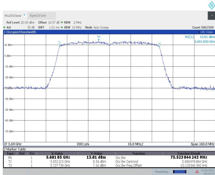
11AC80MIMO_Ant9_5690
