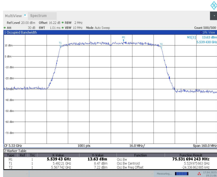
11AC80MIMO_Ant9_5530
