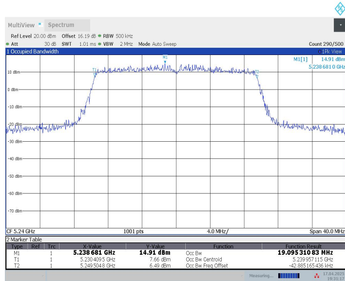
11AX20MIMO_Ant9_5240
