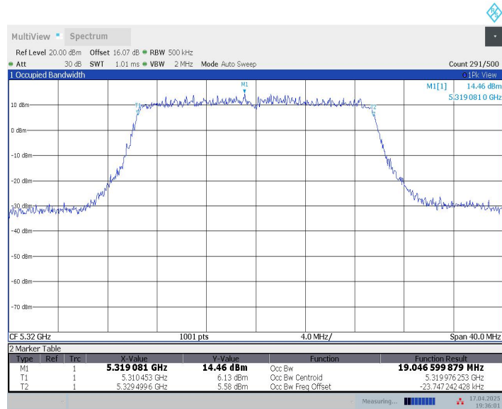
11AX20MIMO_Ant9_5320
