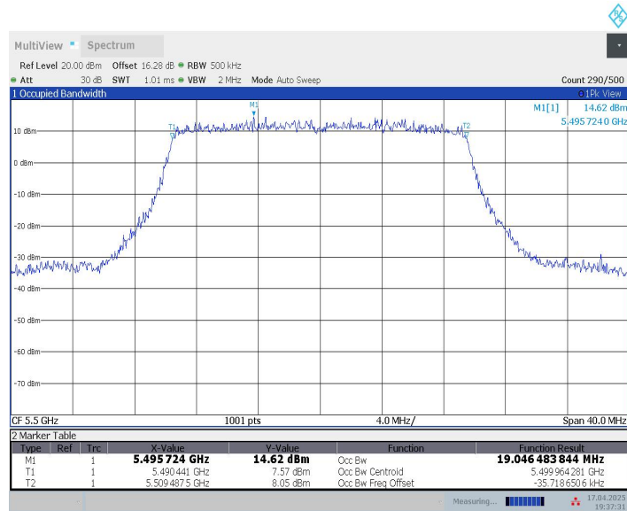
11AX20MIMO_Ant9_5500
