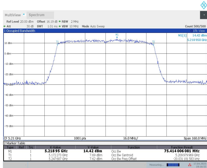
11AC80MIMO_Ant9_5210
