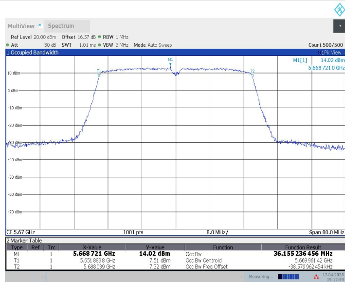
11N40MIMO_Ant9_5670
