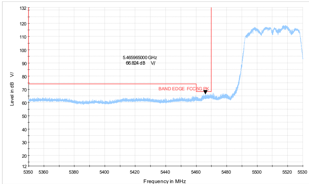
5G WIFI_n40 CH102_5.35-5.53GHz_PK
