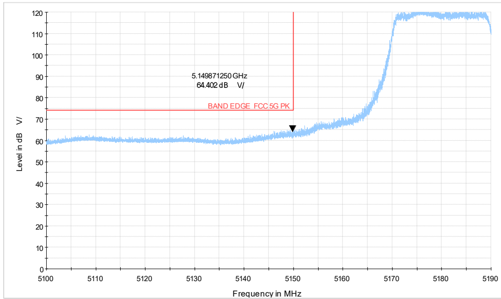
ax20-242TONE_CH36_5.1-5.19GHz_PK
