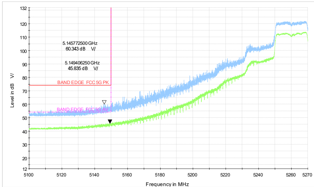
5G WIFI_ax20 CH52_5.1-5.27GHz_MCS0
