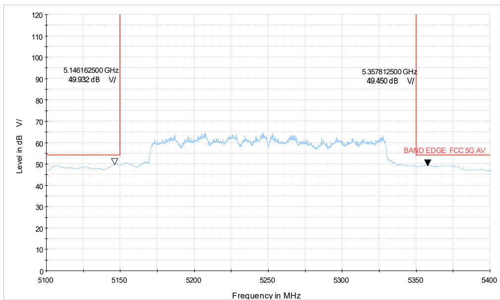
ax160-996x2TONE_CH50_5.1-5.4GHz_AV
