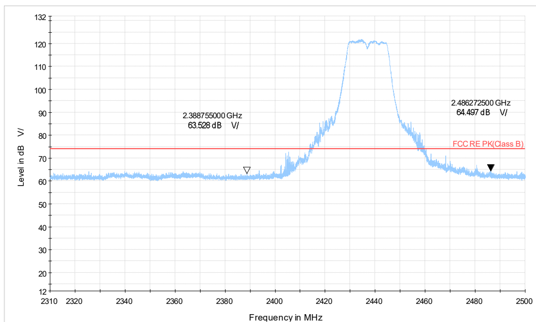
WiFi-2.4Gg_CH6_2.31-2.5GHz_PK
