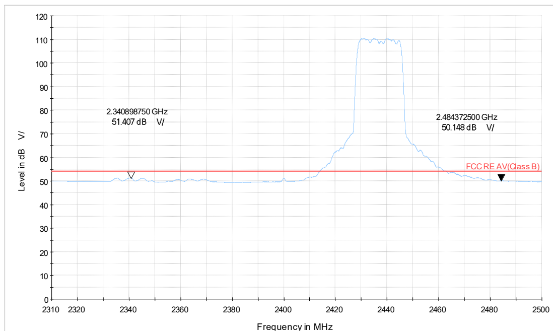
WiFi-2.4Gg_CH6_2.31-2.5GHz_AV
