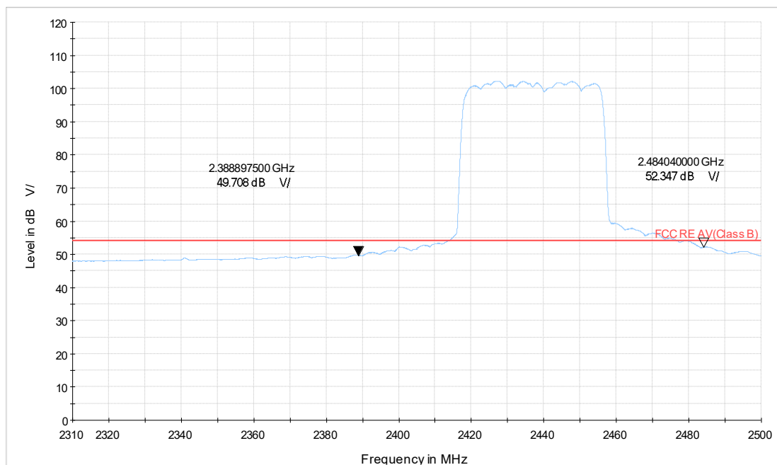
WiFi-2.4Gax40_CH6_2.31-2.5GHz_AV
