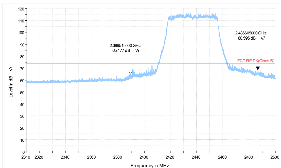
WiFi-2.4Gax40_CH6_2.31-2.5GHz_PK
