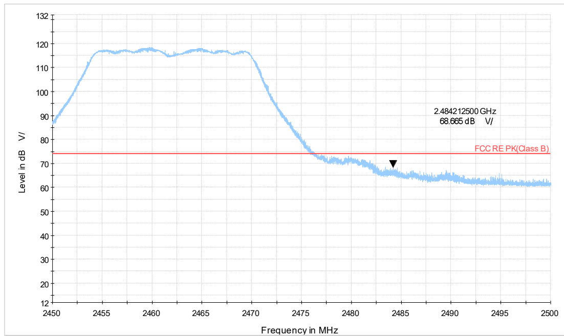
WiFi-2.4Gg_CH11_2.45-2.5GHz_PK
