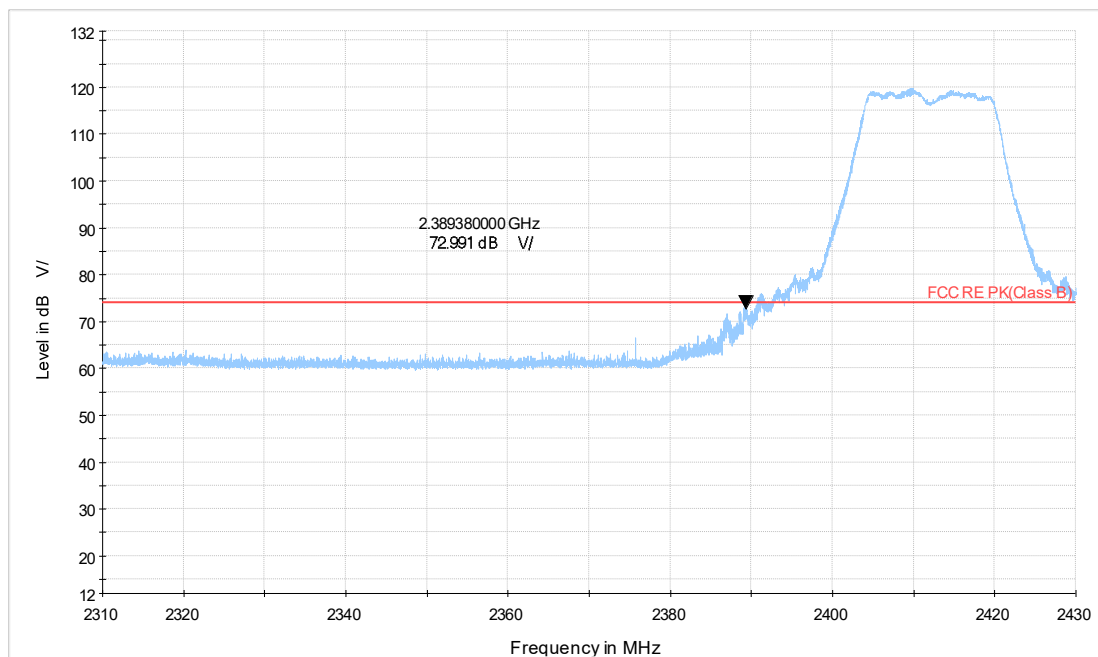
WiFi-2.4Gg_CH1_2.31-2.43GHz_PK
