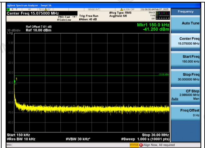
GPRS1900-512-0-0.15~30MHz-PASS
