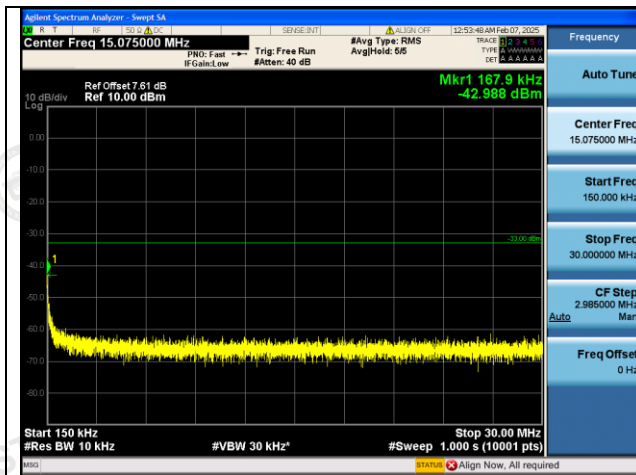
GSM1900-512-0-0.15~30MHz-PASS
