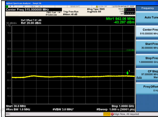
GSM1900-512-0-30~1000MHz-PASS
