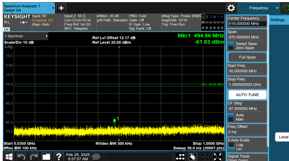
11G-Ant1-2412-30~1000-PASS
