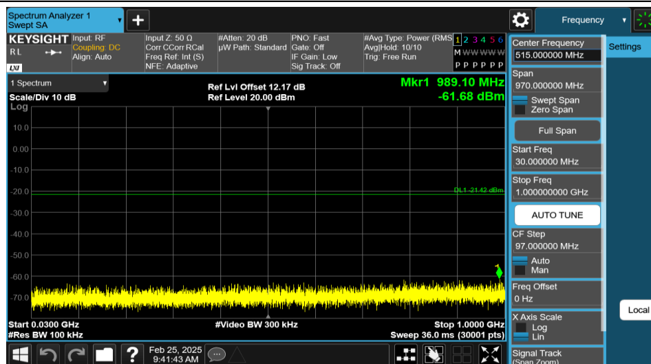
11G-Ant1-2437-30~1000-PASS
