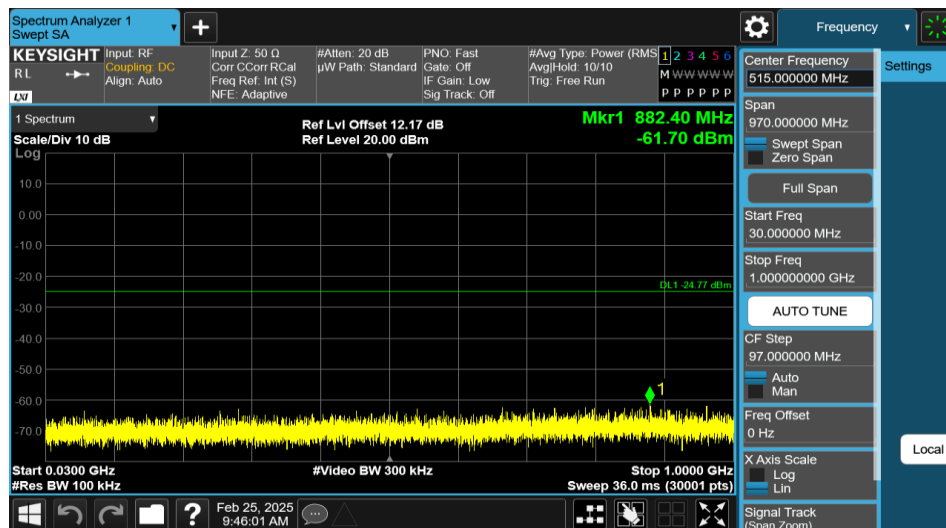
11G-Ant1-2462-30~1000-PASS
