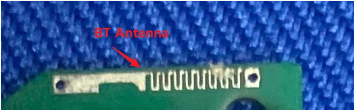
EUT Photo
