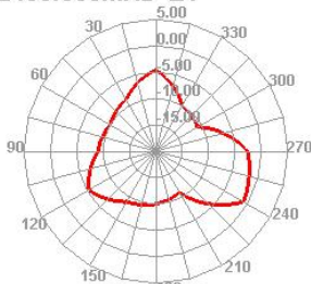
2450.000MHz E1
