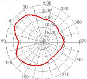
5450.000MHz E1
