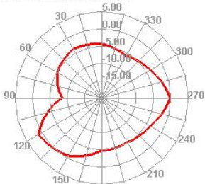
5450.000MHz E2
