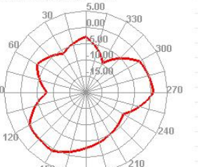
5800.000MHz E2
