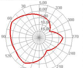
5800.000MHz E1
