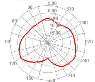
2500.000MHz E2
