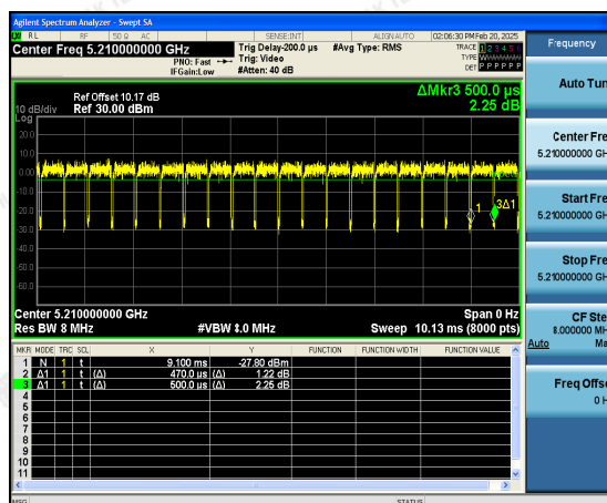
802.11ac(HT80)
