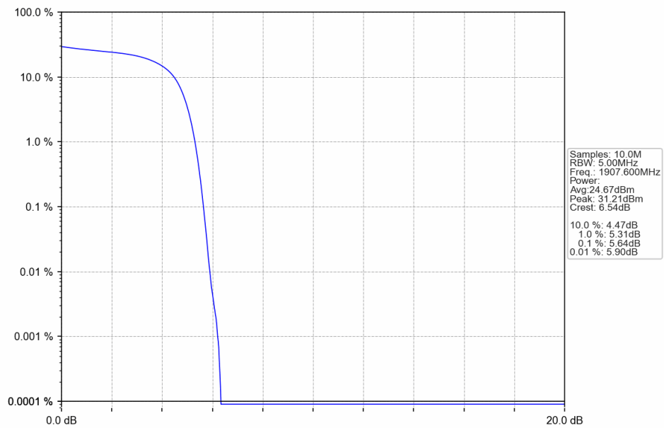
BandII_HSDPA_HCH_1907.6MHz_Subtest 1_NTNV
