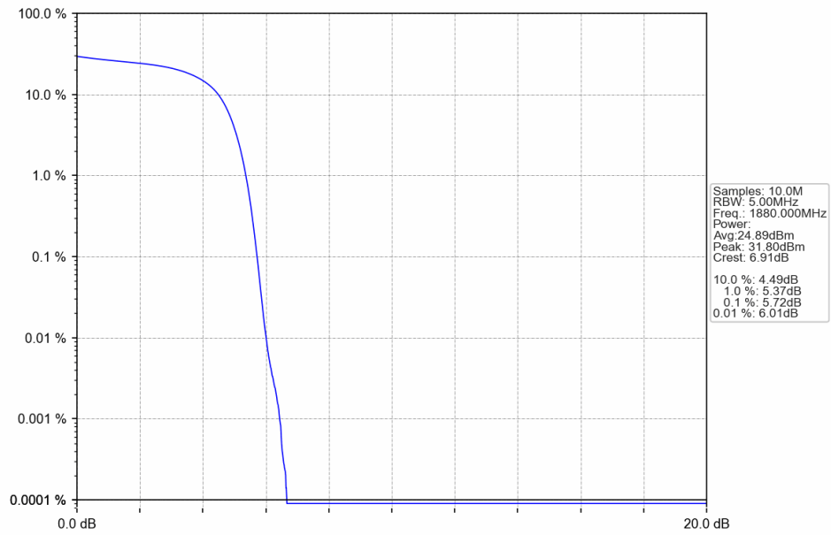
BandII_HSDPA_MCH_1880MHz_Subtest 1_NTNV
