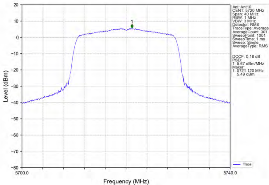
802.11ax(HEW20)_HCH_5720MHz_SU_/_Ant10_NTNV
