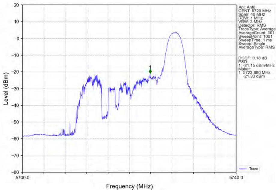
802.11ax(HEW20)_HCH_5720MHz_RU26_Right_Ant8_NTNV
