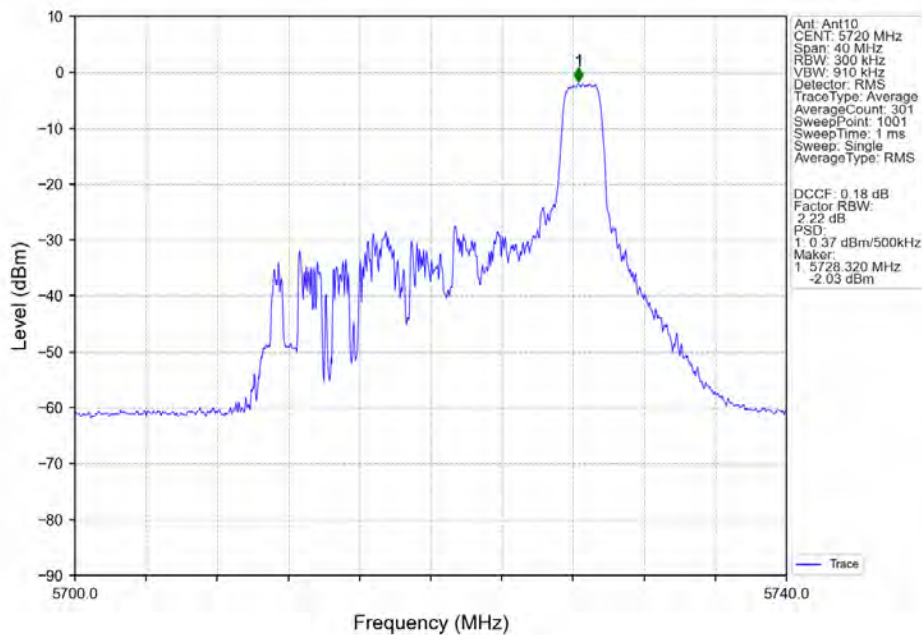
802.11ax(HEW20)_HCH_5720MHz_RU26_Right_Ant10_NTNV
