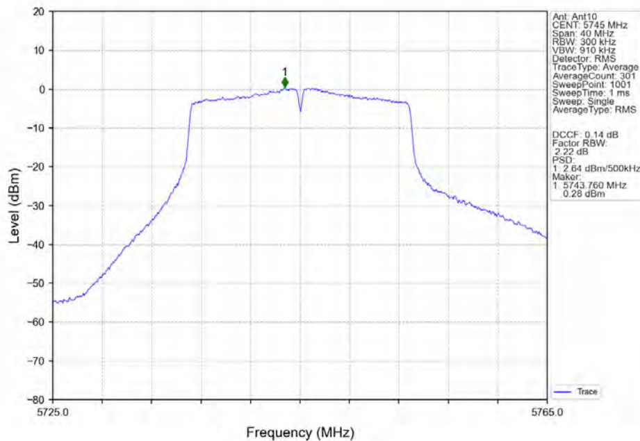
802.11n(HT20)_LCH_5745MHz_Ant10_NTNV
