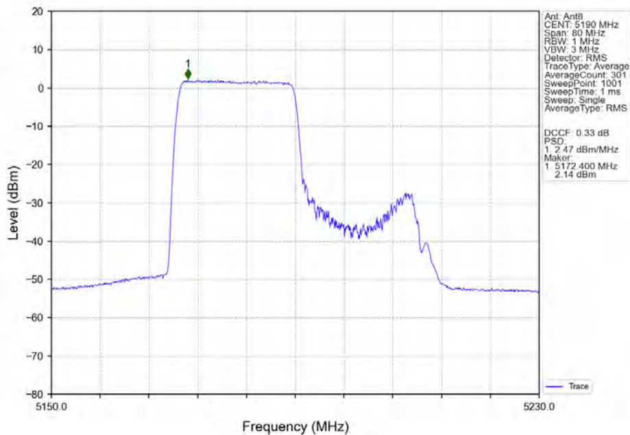
802.11ax(HEW40)_LCH_5190MHz_RU242_Left_Ant8_NTNV
