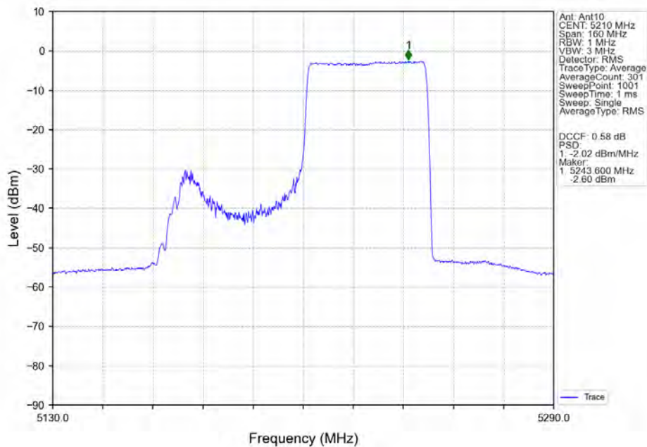
802.11ax(HEW80)_MCH_5210MHz_RU484_Right_Ant10_NTNV
