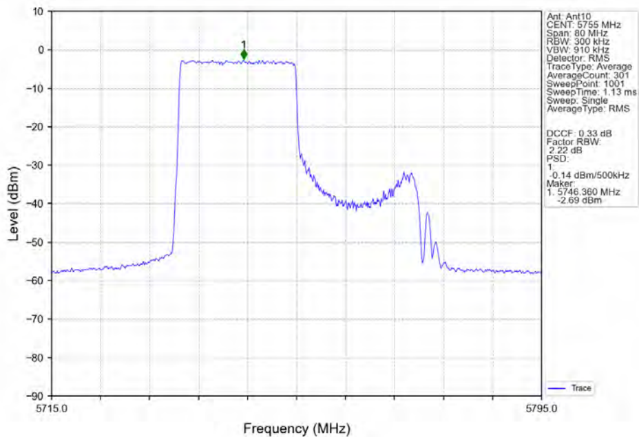
802.11ax(HEW40)_LCH_5755MHz_RU242_Left_Ant10_NTNV
