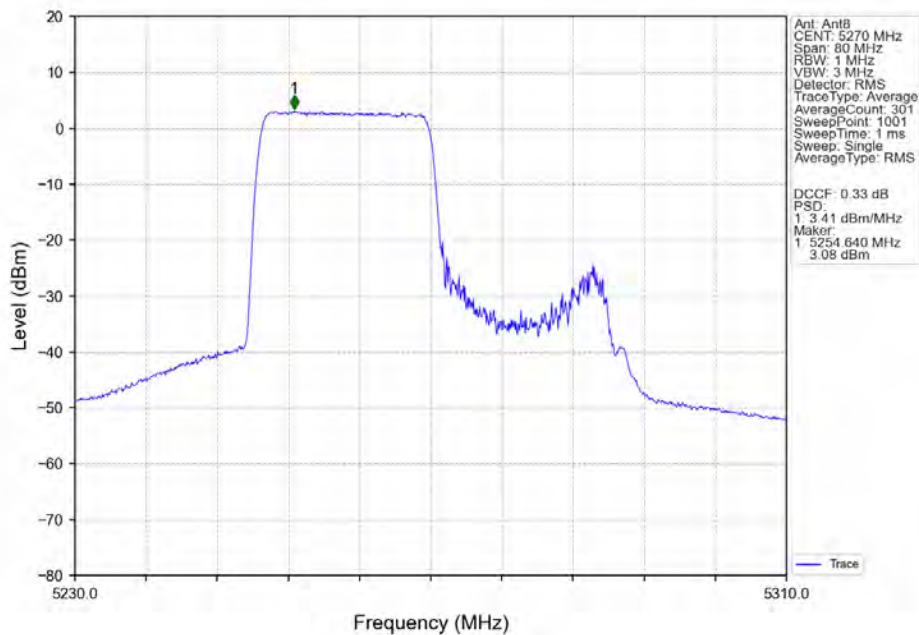
802.11ax(HEW40)_LCH_5270MHz_RU242_Left_Ant8_NTNV
