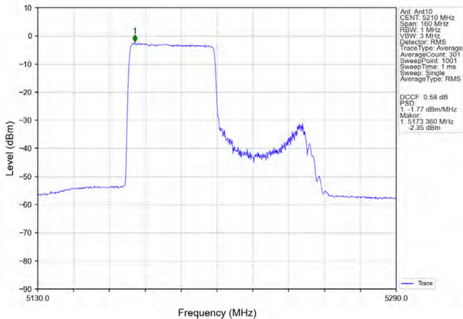
802.11ax(HEW80)_MCH_5210MHz_RU484_Left_MIMO_NTNV
