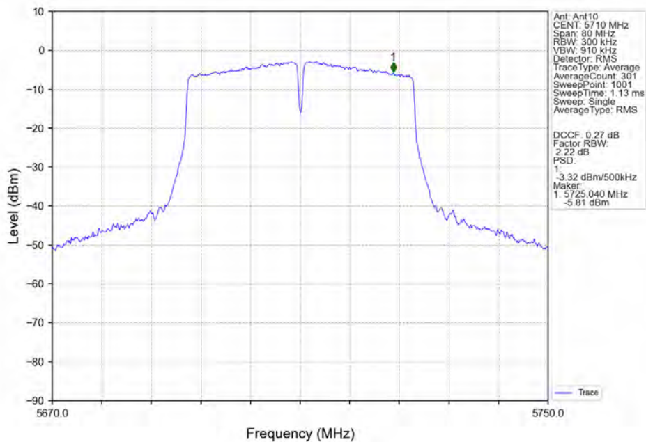
802.11n(HT40)_HCH_5710MHz_Ant10_NTNV
