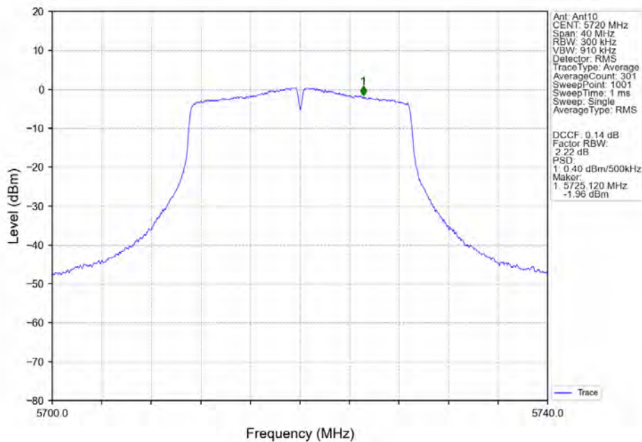
802.11ac(VHT20)_HCH_5720MHz_Ant10_NTNV
