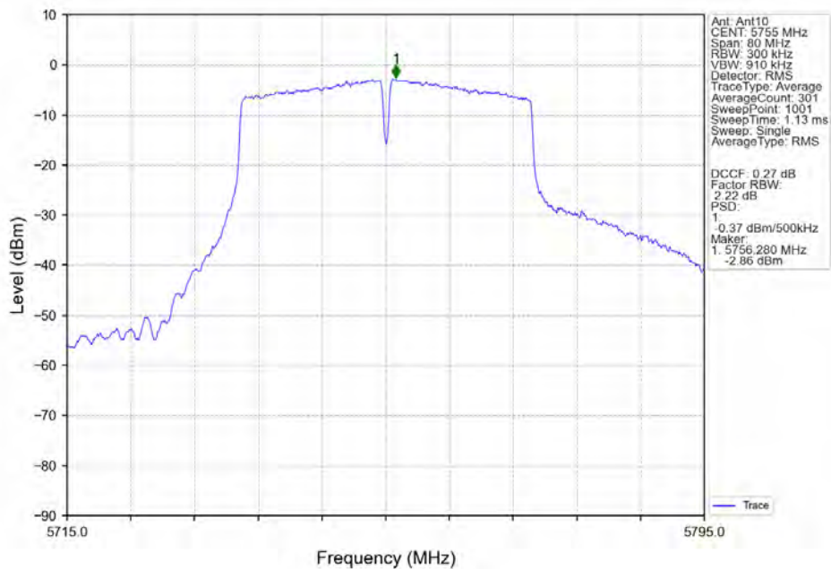
802.11n(HT40)_LCH_5755MHz_Ant10_NTNV
