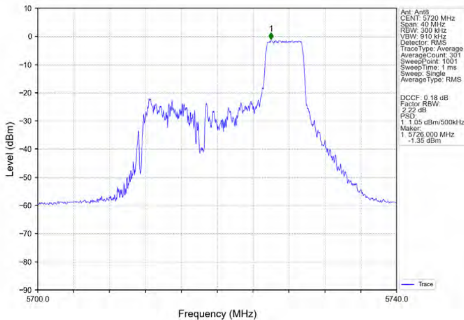
802.11ax(HEW20)_HCH_5720MHz_RU52_Right_Ant8_NTNV
