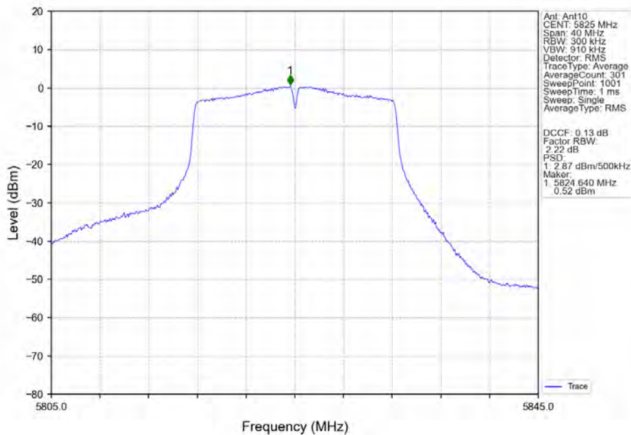
802.11a_HCH_5825MHz_Ant10_NTNV
