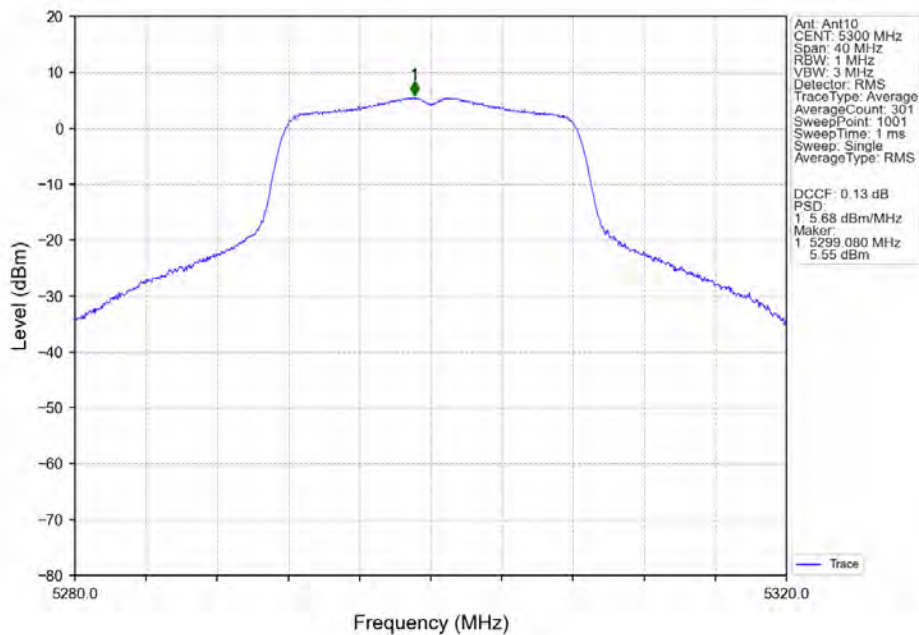
802.11a_MCH_5300MHz_Ant10_NTNV
