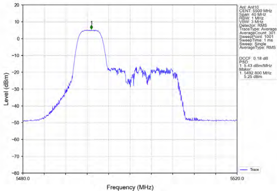
802.11ax(HEW20)_LCH_5500MHz_RU52_Left_Ant10_NTNV
