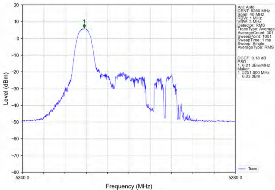
802.11ax(HEW20)_LCH_5260MHz_RU26_Left_Ant8_NTNV
