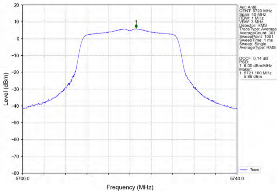
802.11n(HT20)_HCH_5720MHz_Ant8_NTNV
