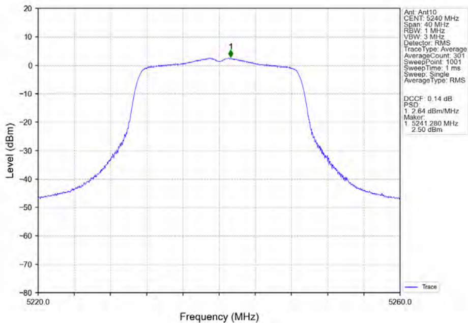
802.11n(HT20)_HCH_5240MHz_Ant10_NTNV
