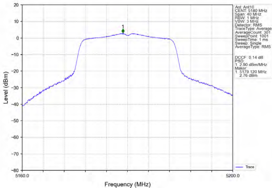
802.11n(HT20)_LCH_5180MHz_Ant10_NTNV
