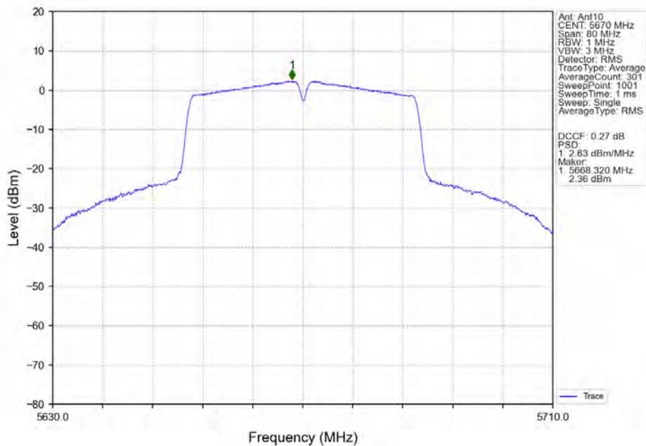
802.11n(HT40)_HCH_5670MHz_Ant10_NTNV
