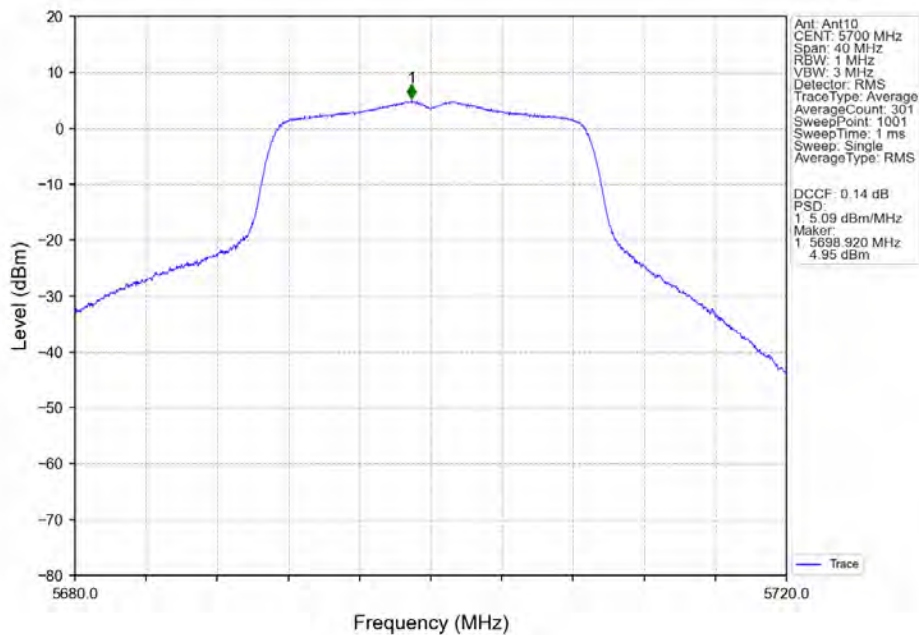
802.11ac(VHT20)_HCH_5700MHz_Ant10_NTNV
