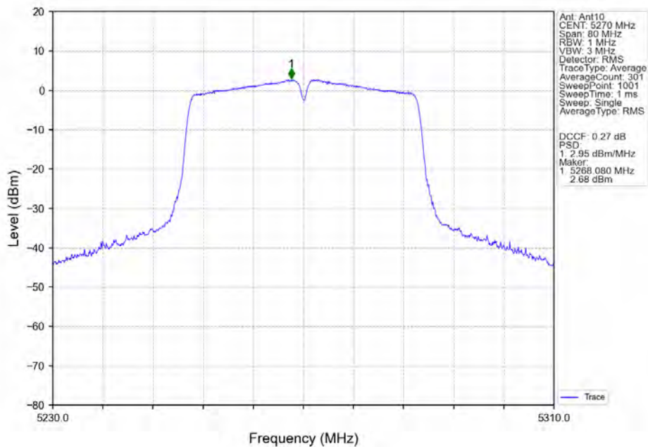
802.11n(HT40)_LCH_5270MHz_Ant10_NTNV
