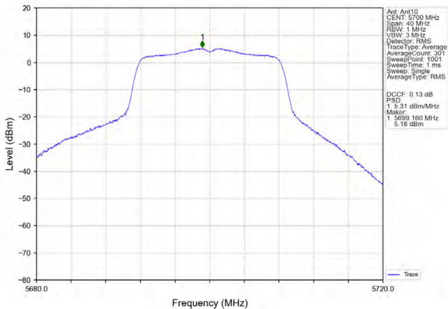
802.11a_HCH_5700MHz_Ant10_NTNV
