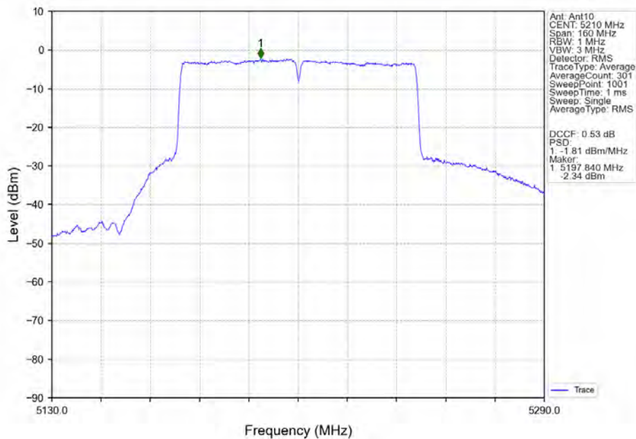
802.11ac(VHT80)_MCH_5210MHz_Ant10_NTNV
