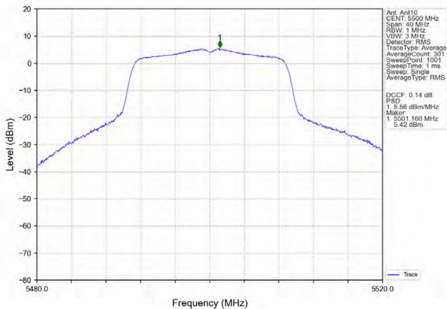
802.11n(HT20)_LCH_5500MHz_Ant10_NTNV
