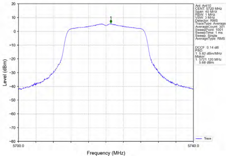
802.11n(HT20)_HCH_5720MHz_MIMO_NTNV
