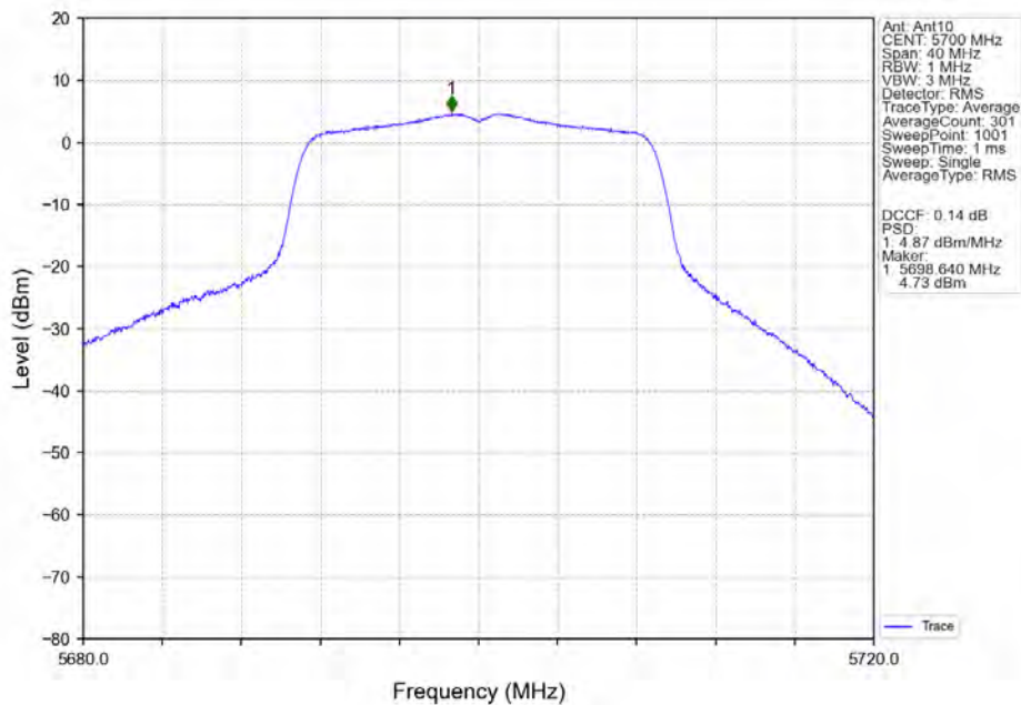
802.11n(HT20)_HCH_5700MHz_Ant10_NTNV
