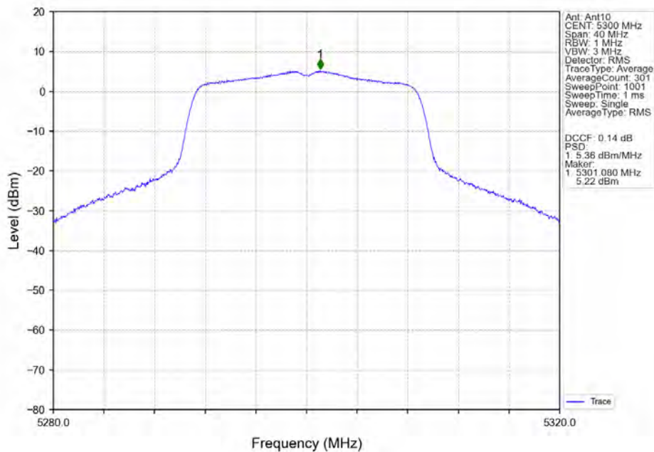
802.11n(HT20)_MCH_5300MHz_Ant10_NTNV
