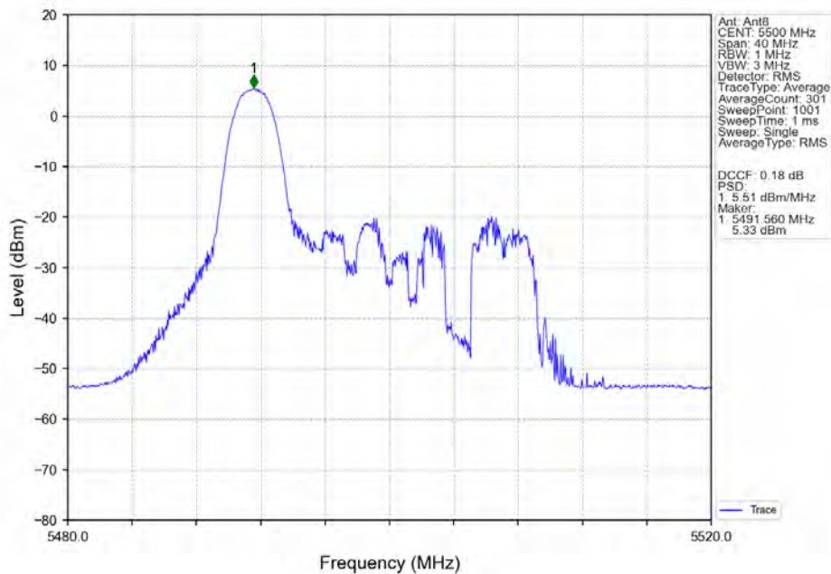
802.11ax(HEW20)_LCH_5500MHz_RU26_Left_Ant8_NTNV
