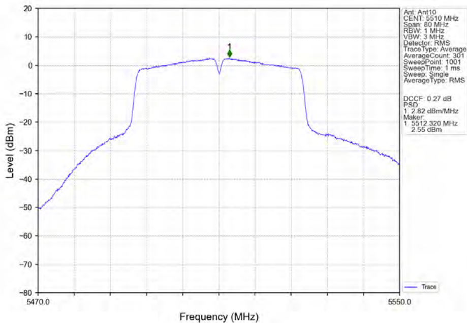
802.11n(HT40)_LCH_5510MHz_Ant10_NTNV
