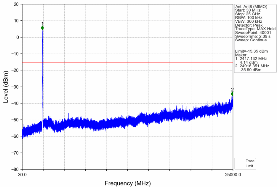
802.11n(HT40)_LCH_2422MHz_Ant8 (MIMO)_NTNV
