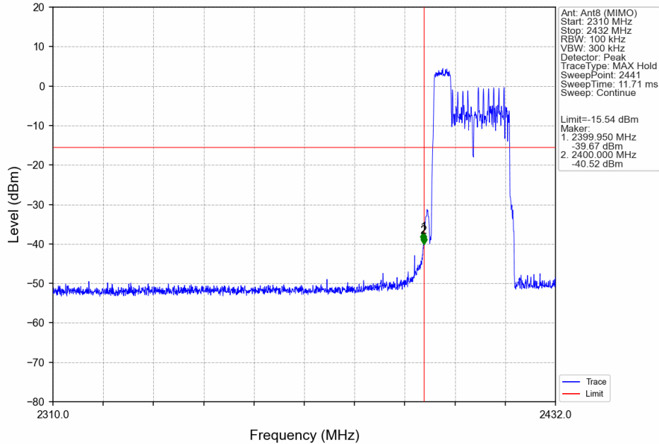
802.11ax(HEW20)_LCH_2412MHz_RU52_Left_Ant8 (MIMO)_NTNV
