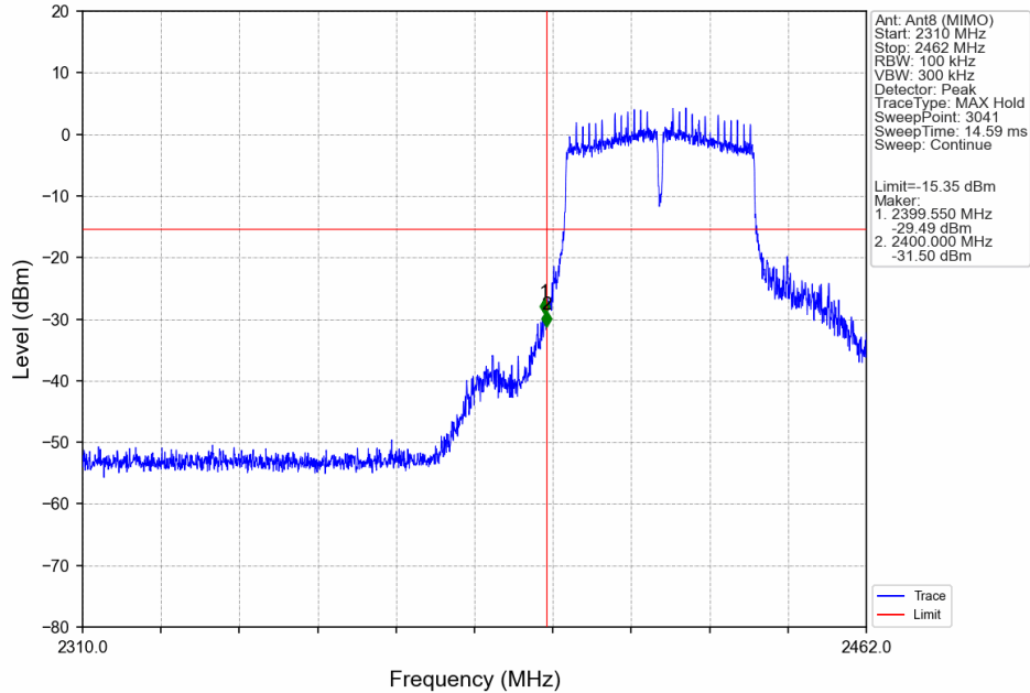
802.11n(HT40)_LCH_2422MHz_Ant8 (MIMO)_NTNV
