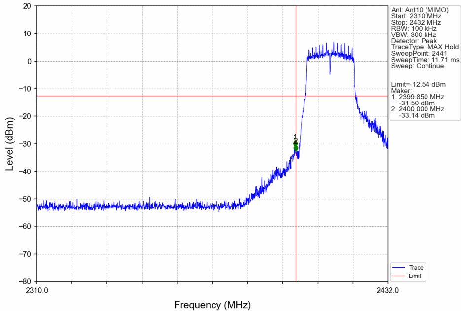
802.11g_LCH_2412MHz_Ant10 (MIMO)_NTNV
