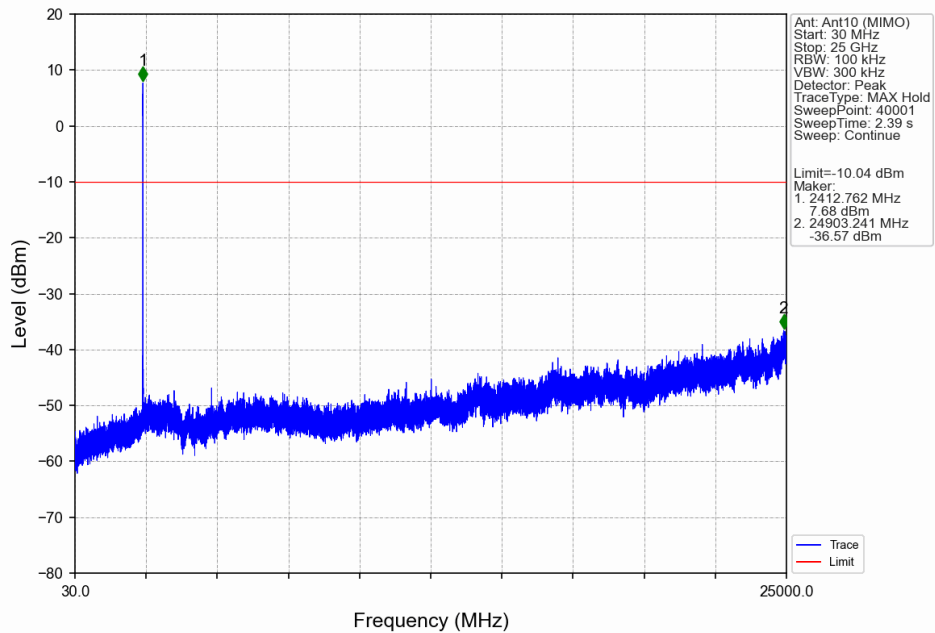
802.11b_LCH_2412MHz_Ant10 (MIMO)_NTNV
