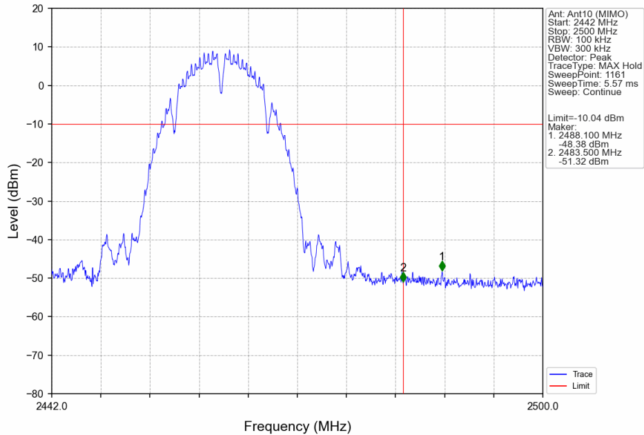
802.11b_HCH_2462MHz_Ant10 (MIMO)_NTNV
