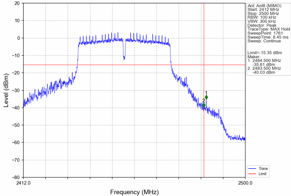
802.11n(HT40)_HCH_2452MHz_Ant8 (MIMO)_NTNV
