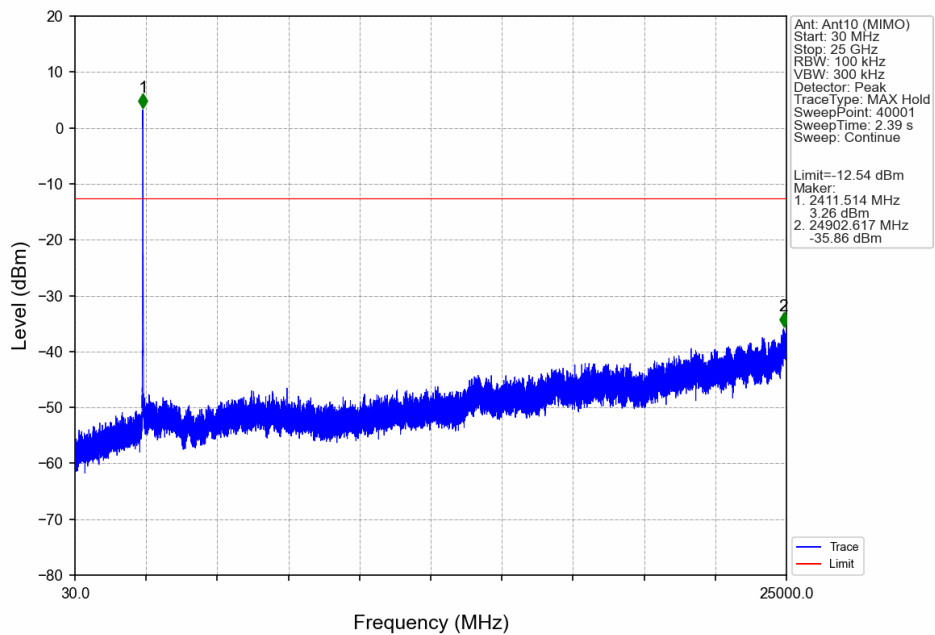
802.11g_LCH_2412MHz_Ant10 (MIMO)_NTNV
