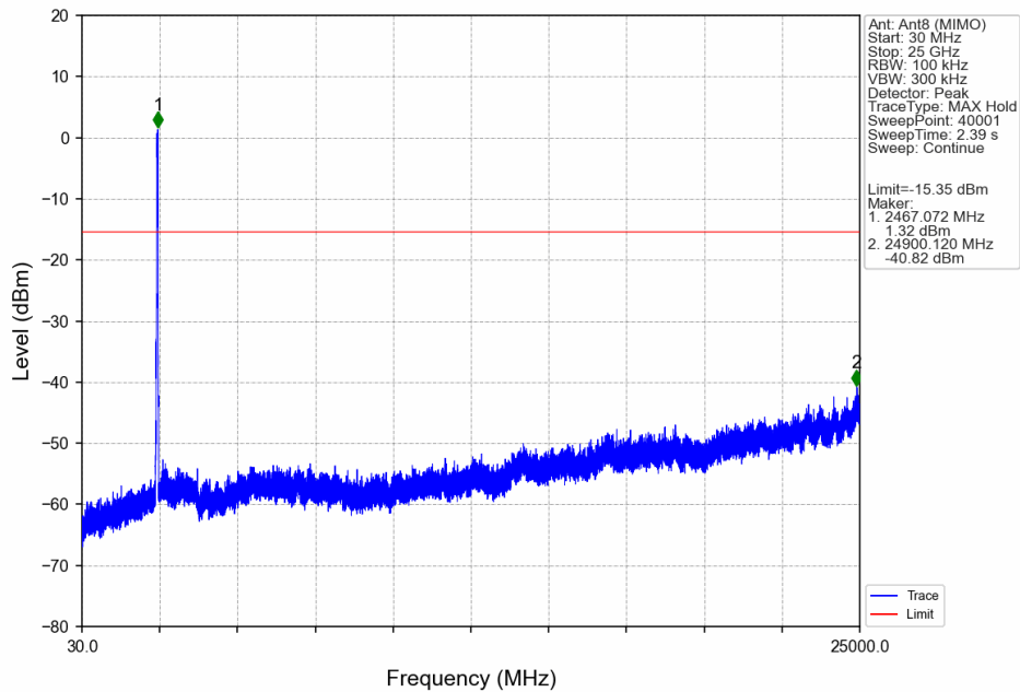
802.11n(HT40)_HCH_2452MHz_Ant8 (MIMO)_NTNV
