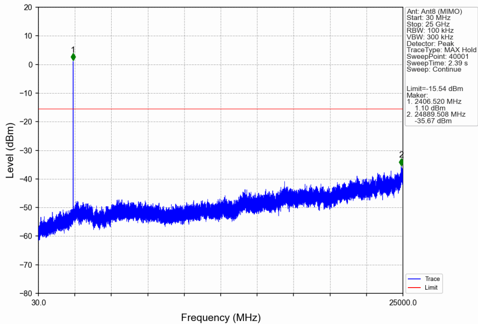
802.11ax(HEW20)_LCH_2412MHz_RU52_Left_Ant8 (MIMO)_NTNV
