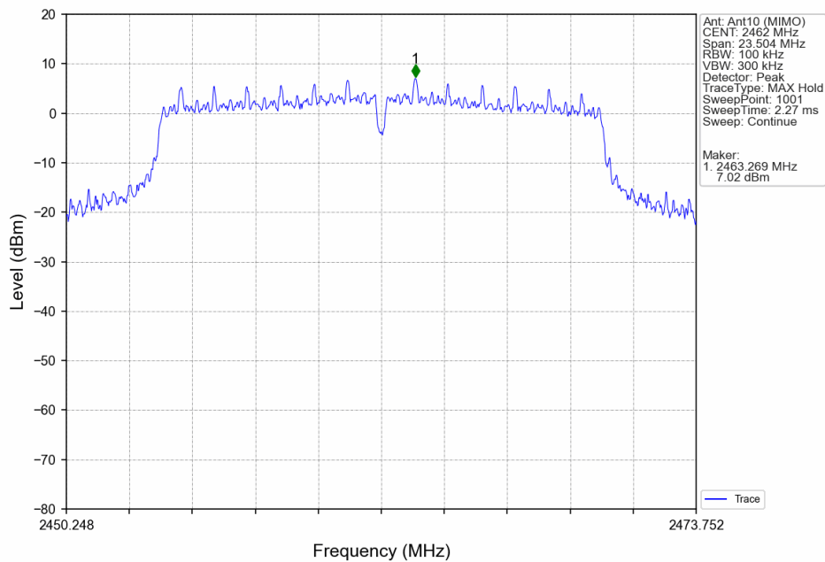
802.11g_HCH_2462MHz_Ant10 (MIMO)_NTNV
