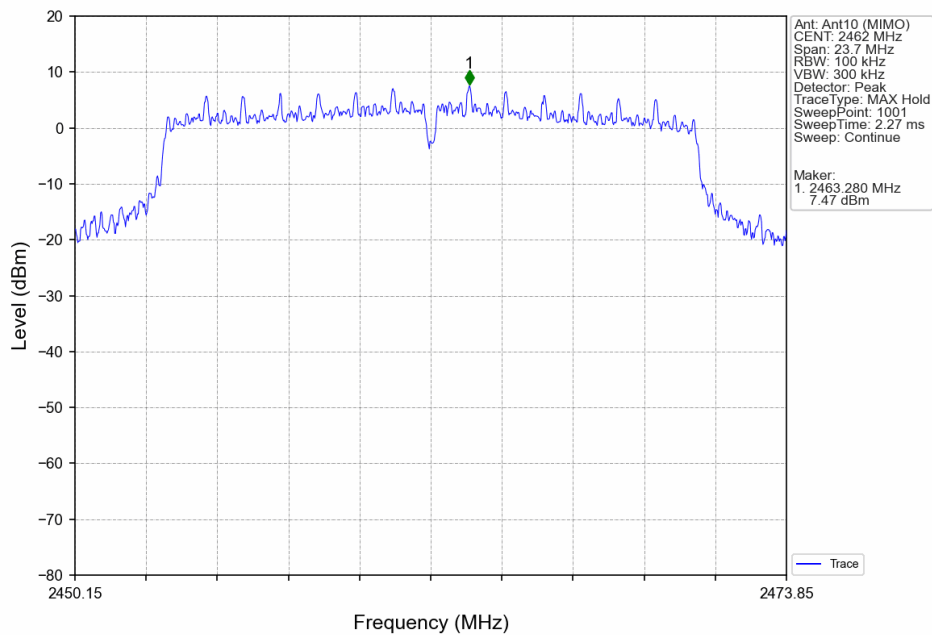
802.11n(HT20)_HCH_2462MHz_Ant10 (MIMO)_NTNV
