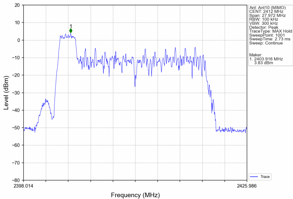
802.11ax(HEW20)_LCH_2412MHz_RU26_Left_Ant10 (MIMO)_NTNV
