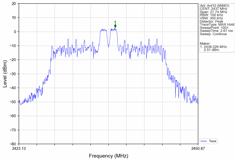
802.11ax(HEW20)_MCH_2437MHz_RU26_Mid_Ant10 (MIMO)_NTNV
