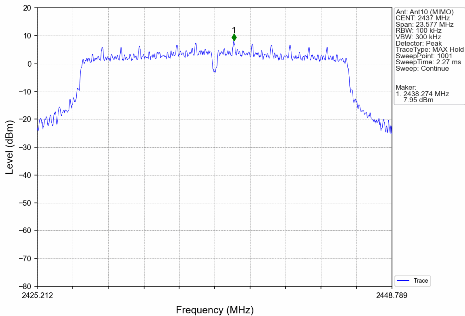
802.11n(HT20)_MCH_2437MHz_Ant10 (MIMO)_NTNV
