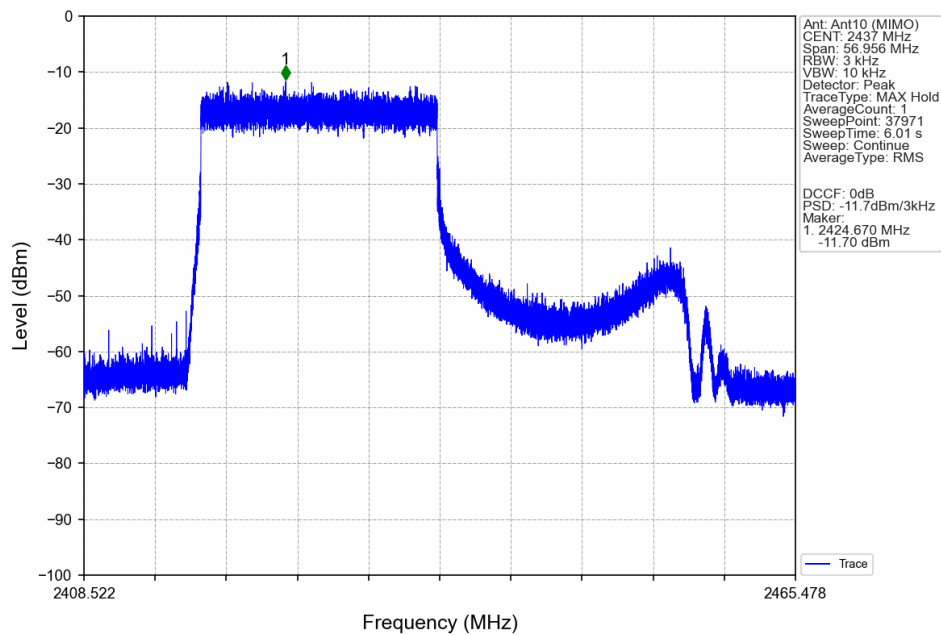
802.11ax(HEW40)_MCH_2437MHz_RU242_Left_Ant10 (MIMO)_NTNV
