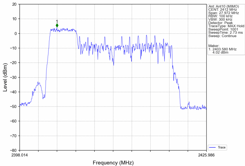
802.11ax(HEW20)_LCH_2412MHz_RU52_Left_Ant10 (MIMO)_NTNV
