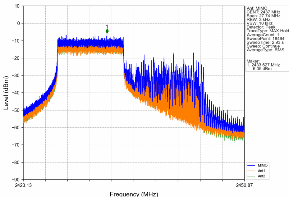
802.11ax(HEW20)_MCH_2437MHz_SU_/_Ant8 (MIMO)_NTNV
