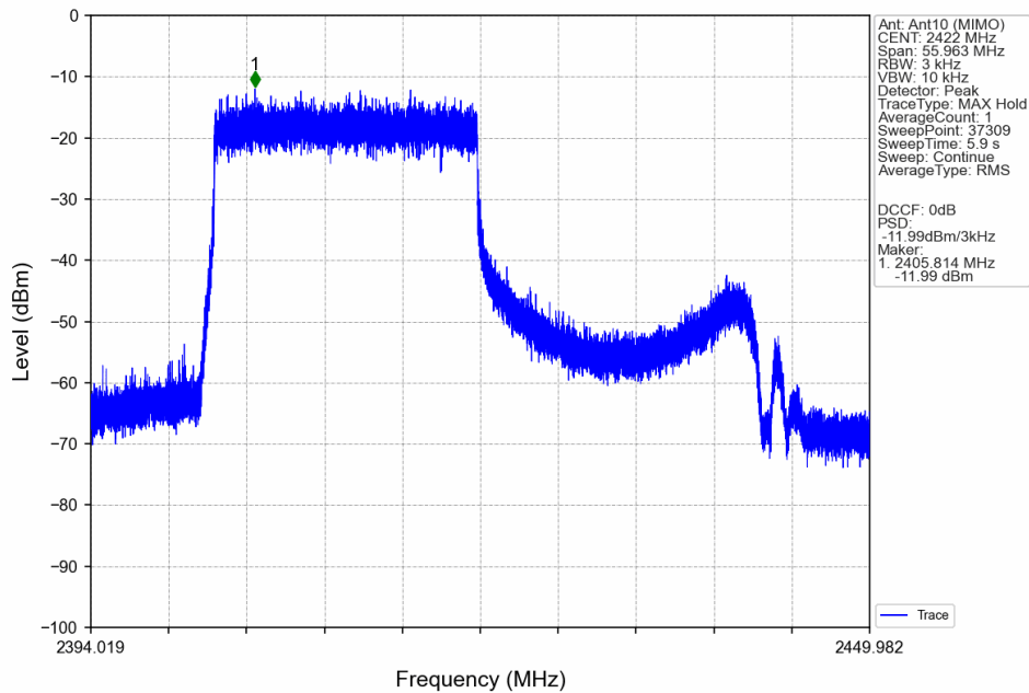
802.11ax(HEW40)_LCH_2422MHz_RU242_Left_Ant10 (MIMO)_NTNV
