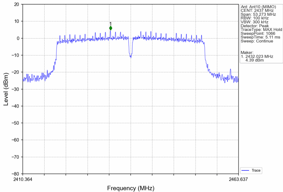
802.11n(HT40)_MCH_2437MHz_Ant10 (MIMO)_NTNV
