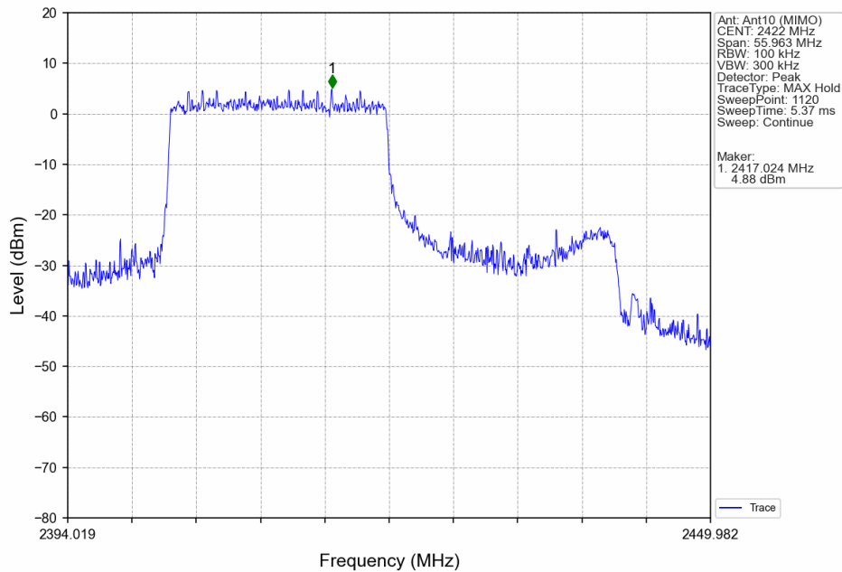
802.11ax(HEW40)_LCH_2422MHz_RU242_Left_Ant10 (MIMO)_NTNV
