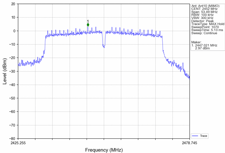
802.11n(HT40)_HCH_2452MHz_Ant10 (MIMO)_NTNV
