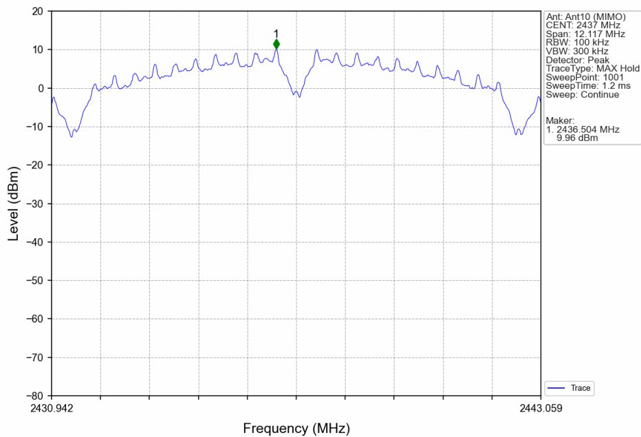
802.11b_MCH_2437MHz_Ant10 (MIMO)_NTNV
