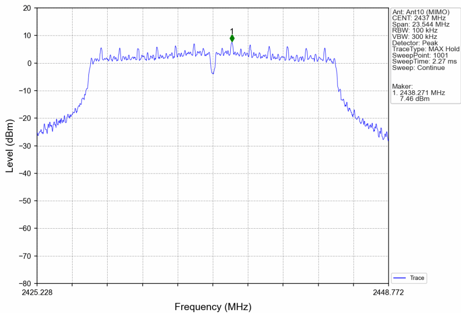
802.11g_MCH_2437MHz_Ant10 (MIMO)_NTNV
