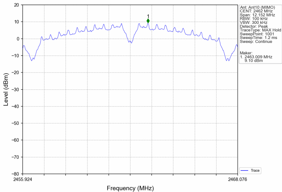
802.11b_HCH_2462MHz_Ant10 (MIMO)_NTNV
