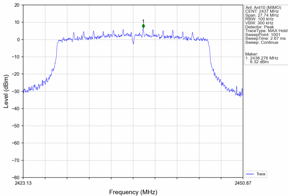
802.11ax(HEW20)_MCH_2437MHz_SU_/_Ant10 (MIMO)_NTNV
