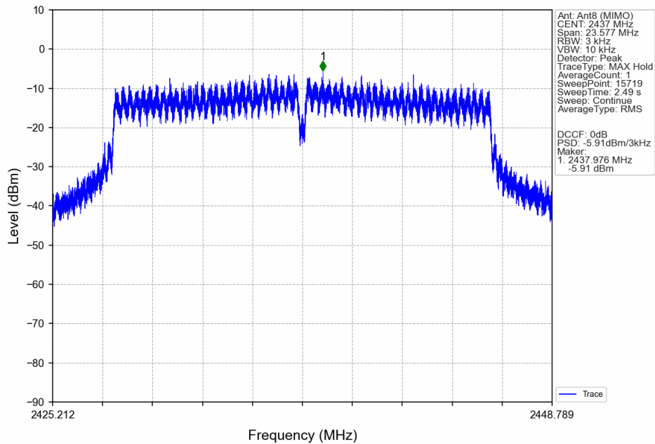
802.11n(HT20)_MCH_2437MHz_Ant8 (MIMO)_NTNV
