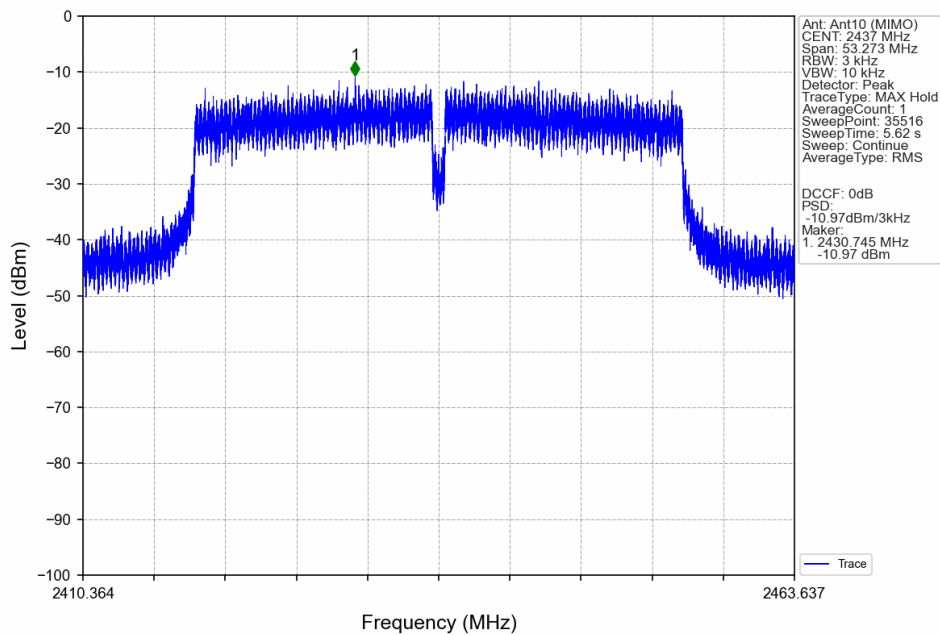
802.11n(HT40)_MCH_2437MHz_Ant10 (MIMO)_NTNV
