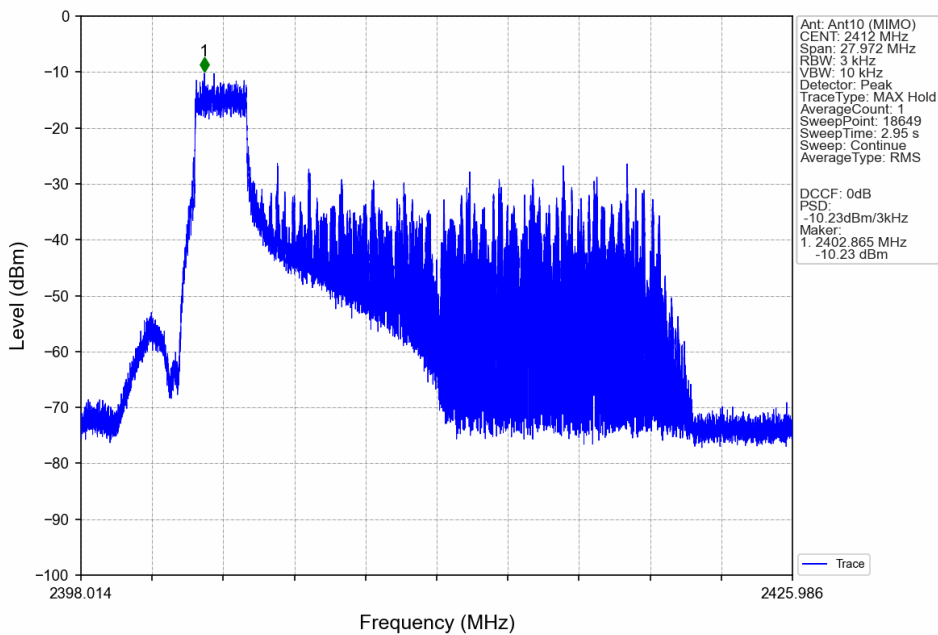
802.11ax(HEW20)_LCH_2412MHz_RU26_Left_Ant10 (MIMO)_NTNV
