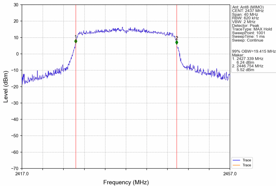
802.11ax(HEW20)_MCH_2437MHz_SU_/_Ant8 (MIMO)_NTNV
