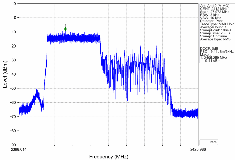
802.11ax(HEW20)_LCH_2412MHz_RU106_Left_Ant10 (MIMO)_NTNV
