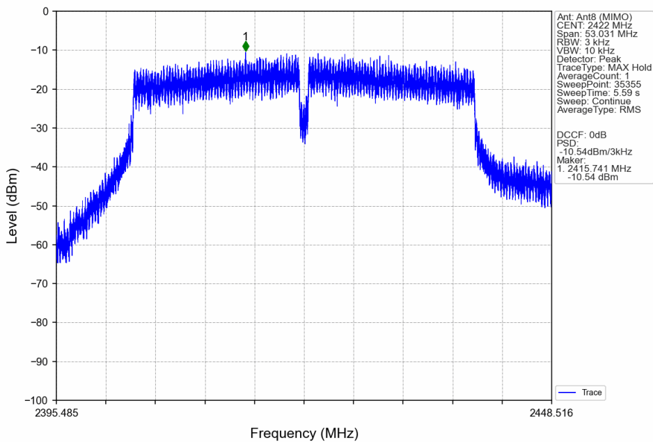
802.11n(HT40)_LCH_2422MHz_Ant8 (MIMO)_NTNV
