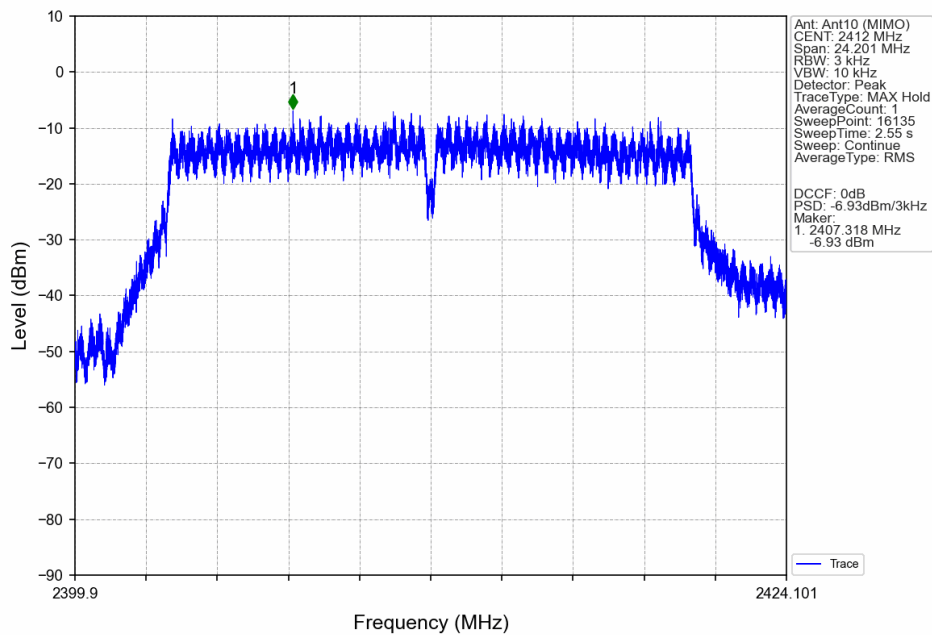
802.11n(HT20)_LCH_2412MHz_Ant10 (MIMO)_NTNV
