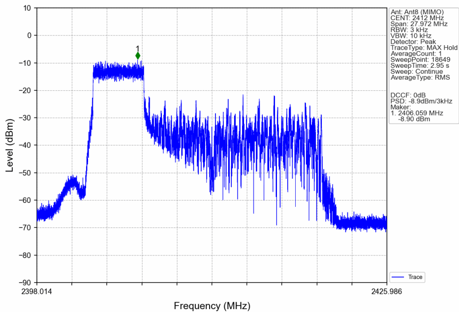
802.11ax(HEW20)_LCH_2412MHz_RU52_Left_Ant8 (MIMO)_NTNV
