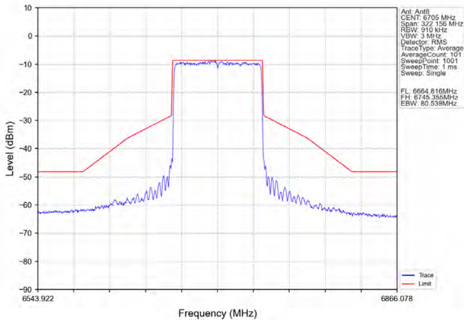
802.11ax(HEW80)_MCH_6705MHz_SU / Ant8_NTNV
