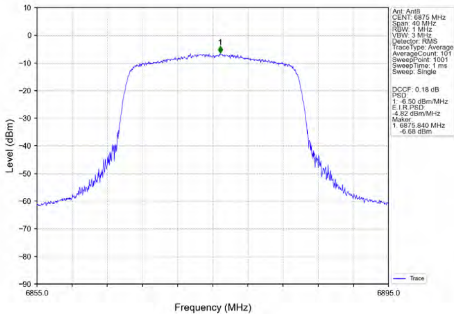
802.11ax(HEW20) HCH 6875MHz SU / Ant8 NTN
