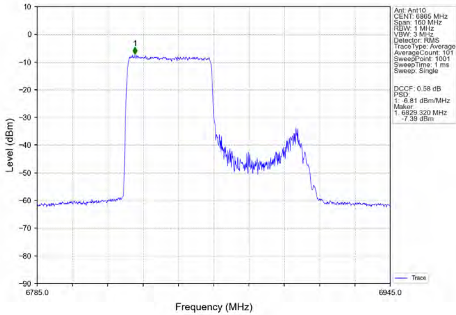
802.11ax(HEW80)_HCH_6865MHz_RU484_Left MIMO NTN
