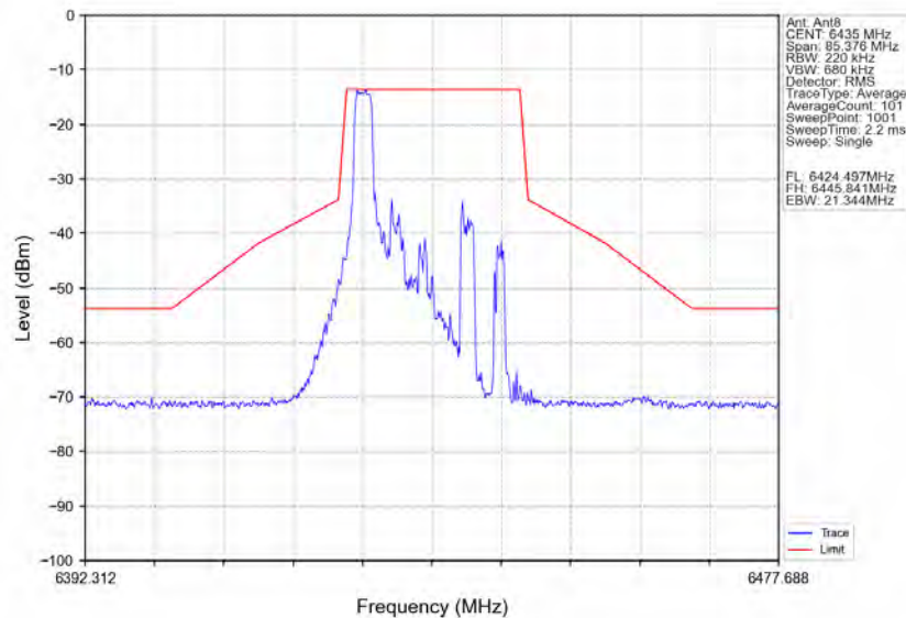
802.11ax(HEW20) LCH 6435MHz RU52 Left Ant8 NTV
