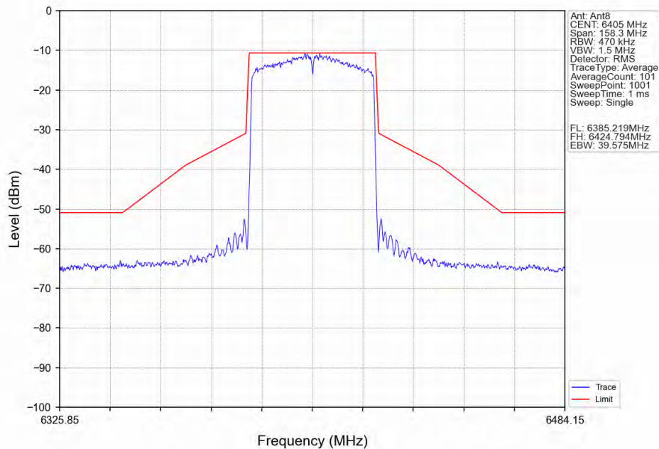
802.11ax(HEW40) HCH 6405MHz SU / Ant8 NTN
