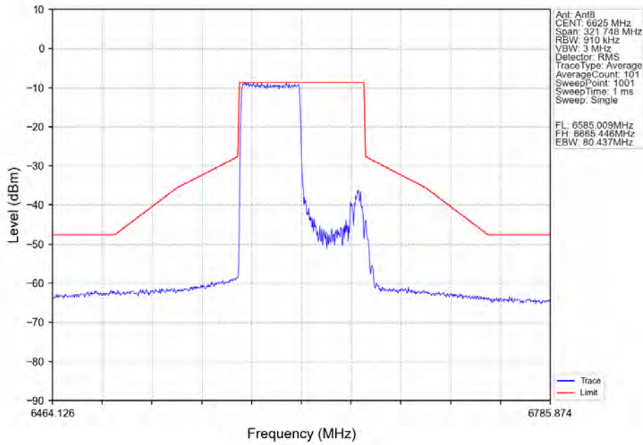
802.11ax(HEW80)_LCH_6625MHz_SU / Ant8_NTNV
