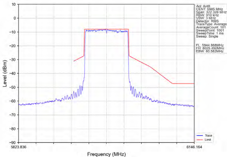
802.11ax(HEW80)_LCH_5985MHz_SU / Ant8_NTNV
