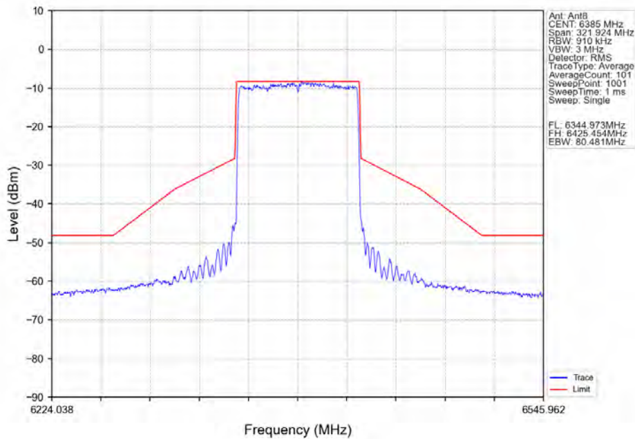
802.11ax(HEW80)_HCH_6385MHz_SU / Ant8_NTNV
