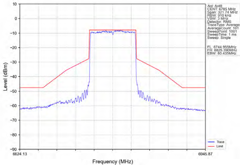
802.11ax(HEW80)_HCH_6785MHz_SU / Ant8_NTNV
