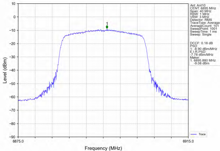
802.11ax(HEW20)_LCH_6895MHz_SU / _Ant10_NTNV
