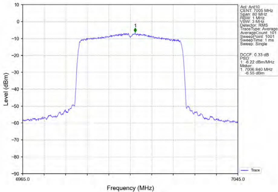
802.11ax(HEW40) MCH 7005MHz SU / Ant10 NTN
