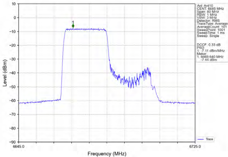
802.11ax(HEW40)_MCH_6685MHz_RU242_Left_Ant10_NTNV
