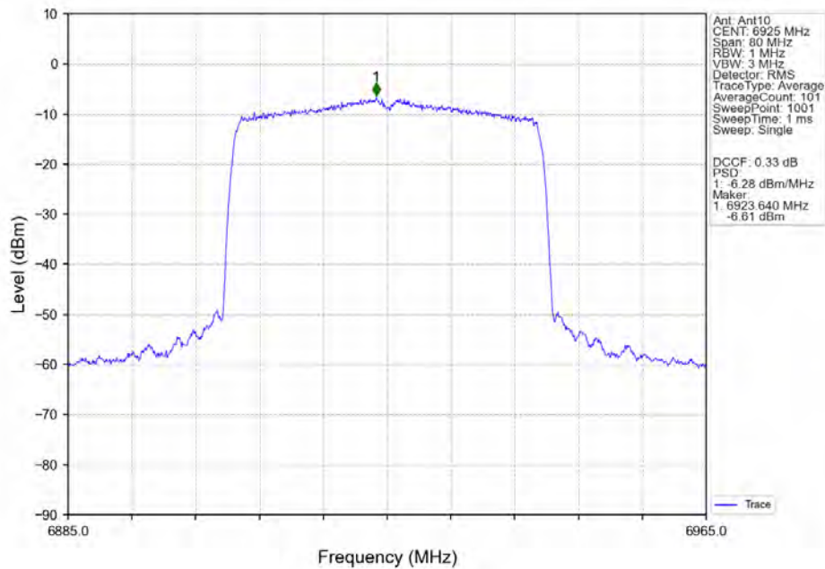
802.11ax(HEW40)_LCH_6925MHz_SU / _Ant10_NTNV
