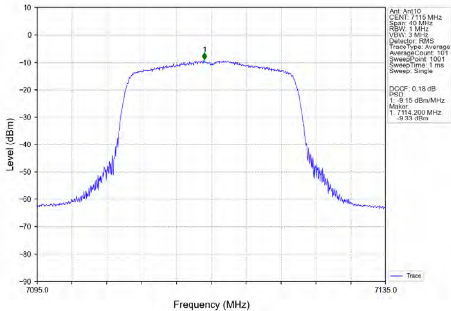
802.11ax(HEW20) HCH 7115MHz SU / Ant10 NTN
