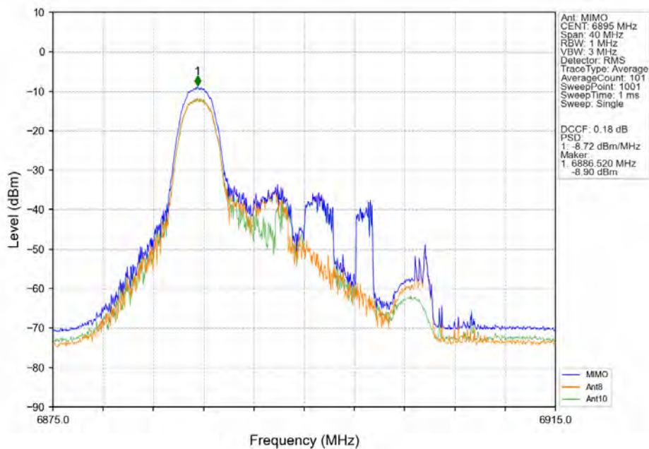
802.11ax(HEW20) LCH 6895MHz RU26 Left MIMO NTN
