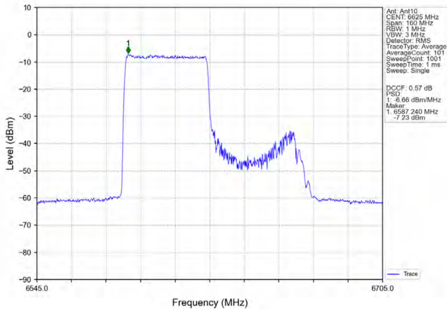
802.11ax(HEW80)_LCH_6625MHz_RU484_Left_Ant10_NTNV
