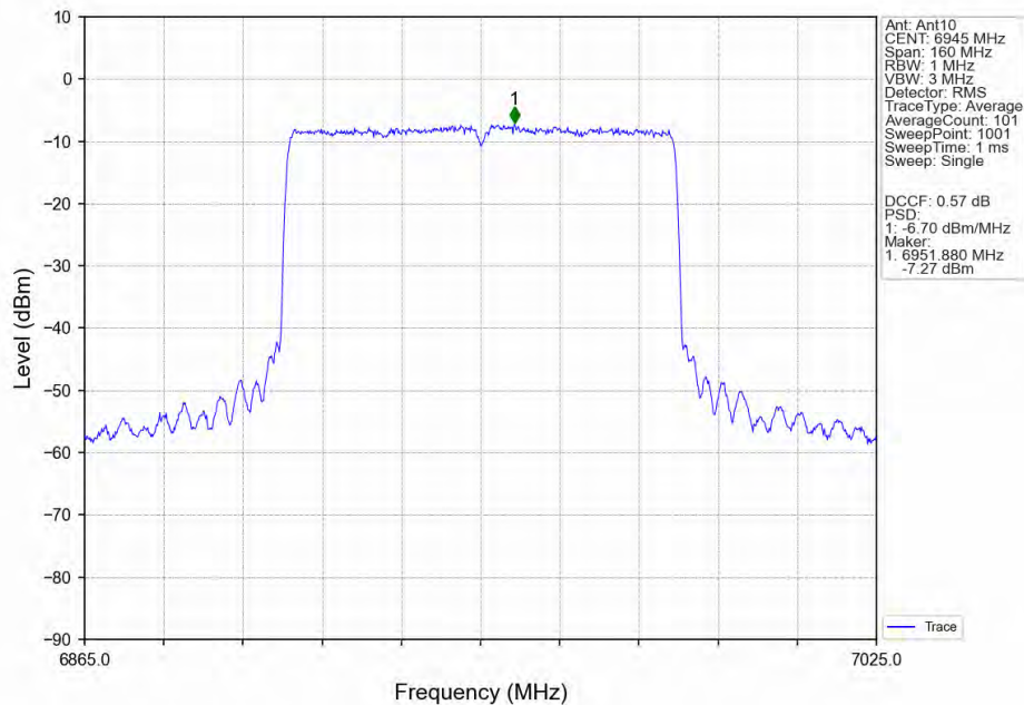
802.11ax(HEW80)_LCH_6945MHz_SU / _Ant10_NTNV
