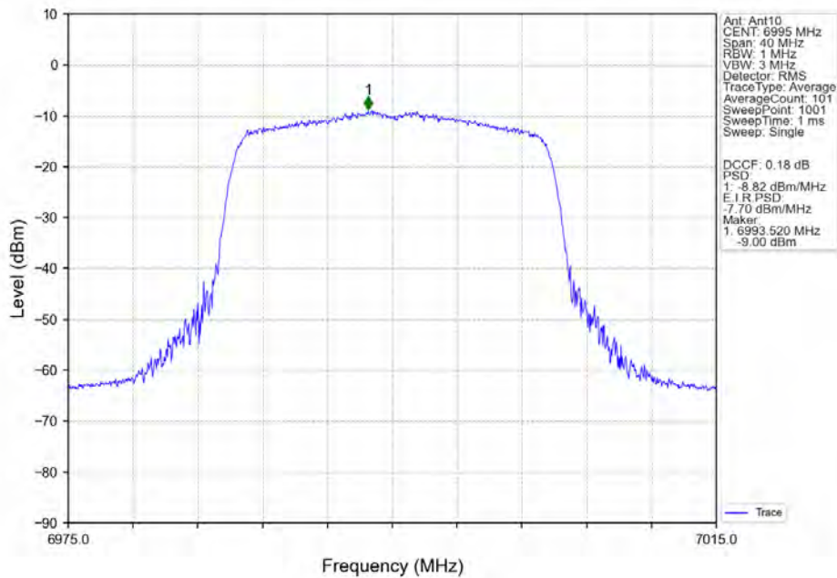
802.11ax(HEW20) MCH 6995MHz SU / Ant10 NTN
