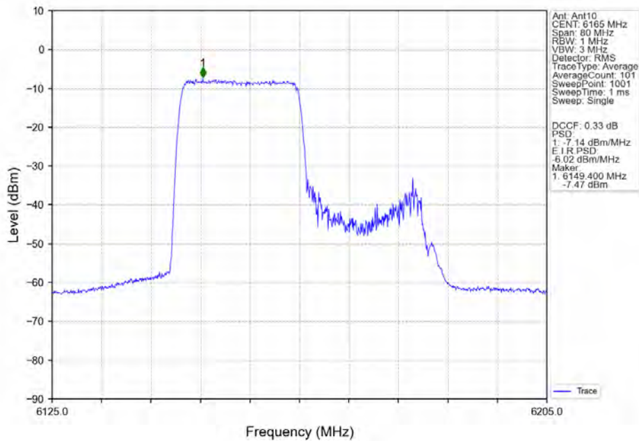
802.11ax(HEW40)_MCH_6165MHz_RU242_Left_Ant10_NTNV
