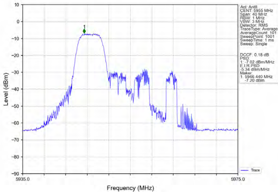
802.11ax(HEW20)_LCH_5955MHz_RU52_Left_Ant8_NTNV
