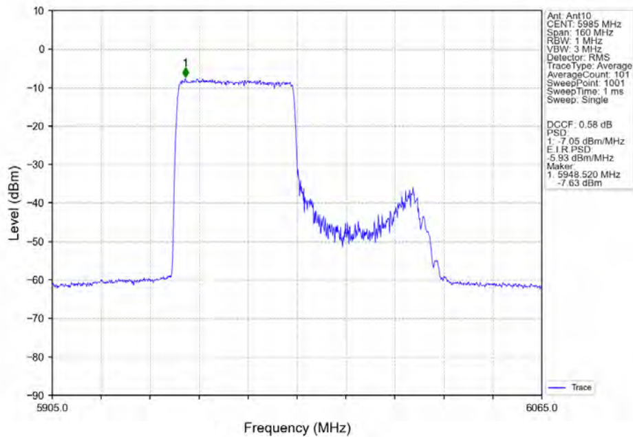
802.11ax(HEW80)_LCH_5985MHz_RU484_Left_Ant10_NTNV
