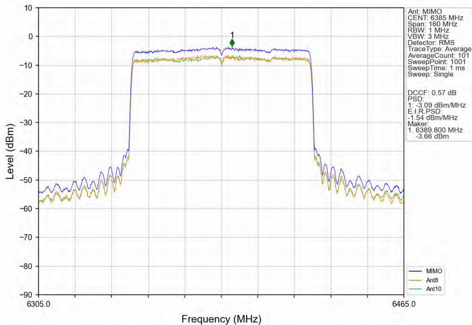
802.11ax(HEW80)_HCH_6385MHz_SU_/_MIMO_NTNV
