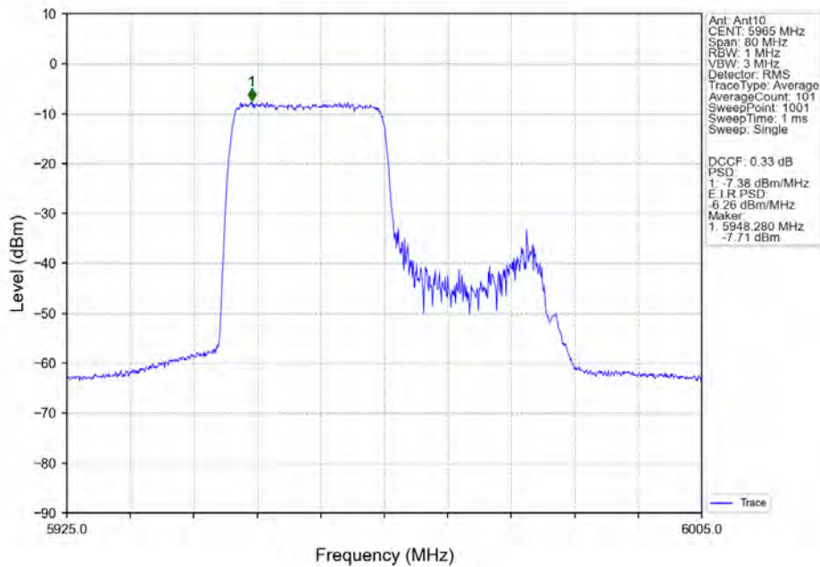
802.11ax(HEW40)_LCH_5965MHz_RU242_Left_Ant10_NTNV
