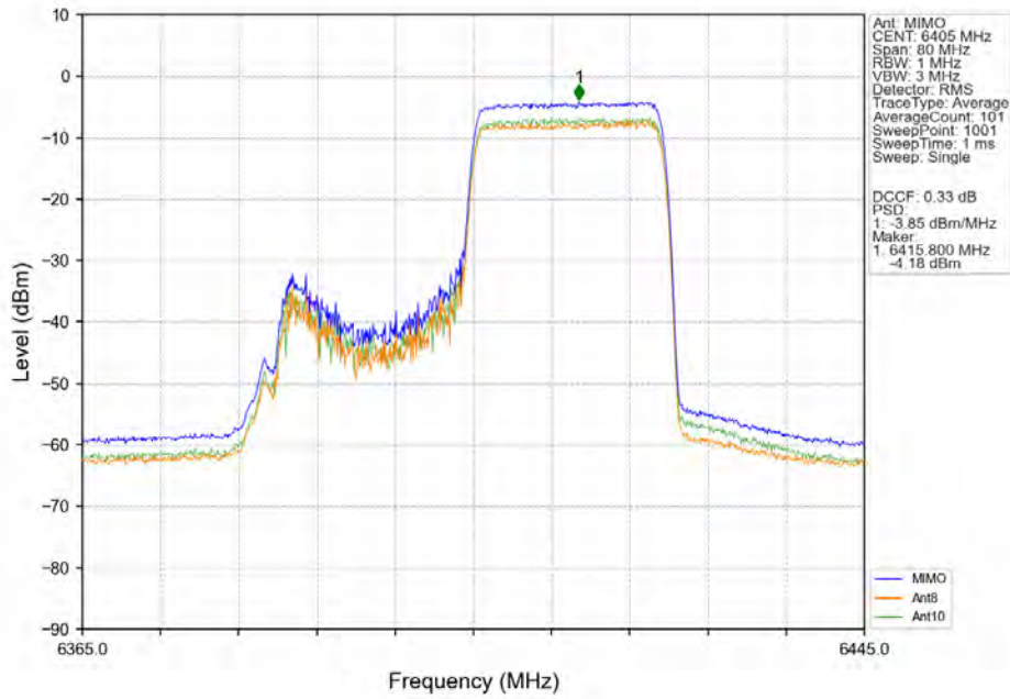
802.11ax(HEW40) HCH 6405MHz SU / Ant8 NTN
