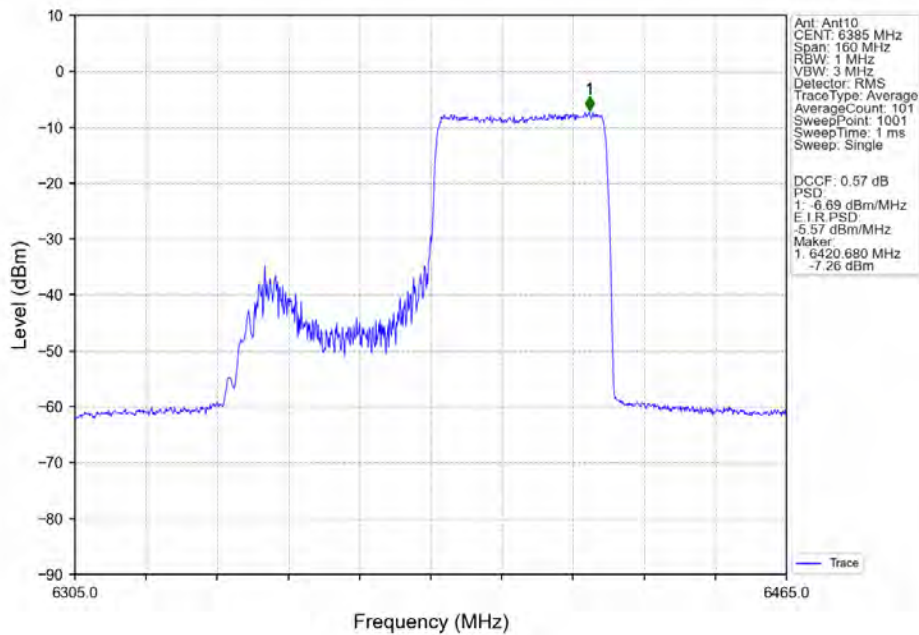
802.11ax(HEW80)_HCH_6385MHz_RU484_Right_Ant10_NTNV
