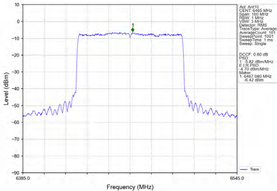
802.11ax(HEW80)_LCH_6465MHz_SU / _Ant10_NTNV
