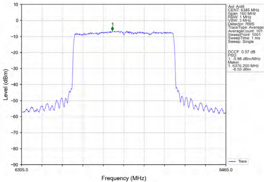
802.11ax(HEW80) HCH 6385MHz SU / Ant8 NTN
