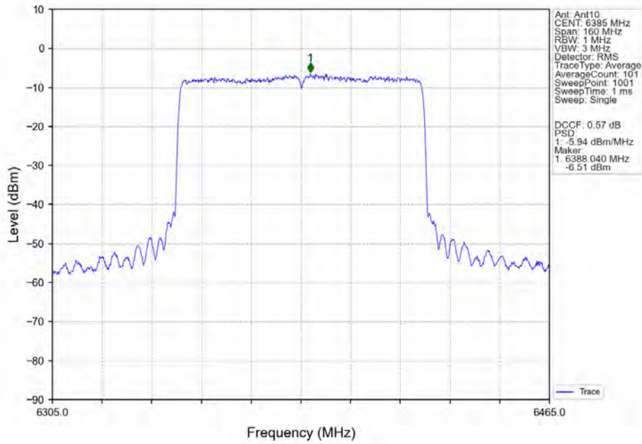
802.11ax(HEW80)_HCH_6385MHz_SU_/_MIMO_NTNV
