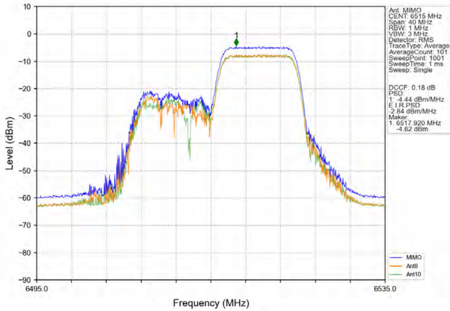
802.11ax(HEW20) HCH 6515MHz SU / Ant8 NTN
