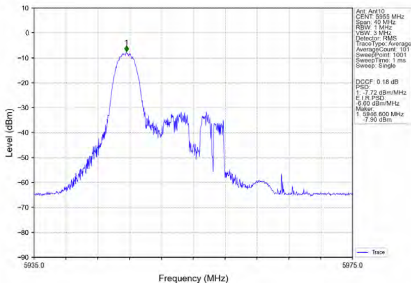
802.11ax(HEW20) LCH 5955MHz RU26 Left Ant10 NTN
