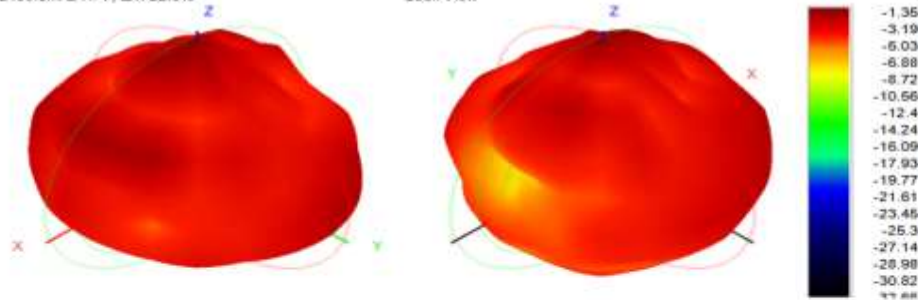
2450.0MHz Total(E2-YZ), Max=-3.08dBi
