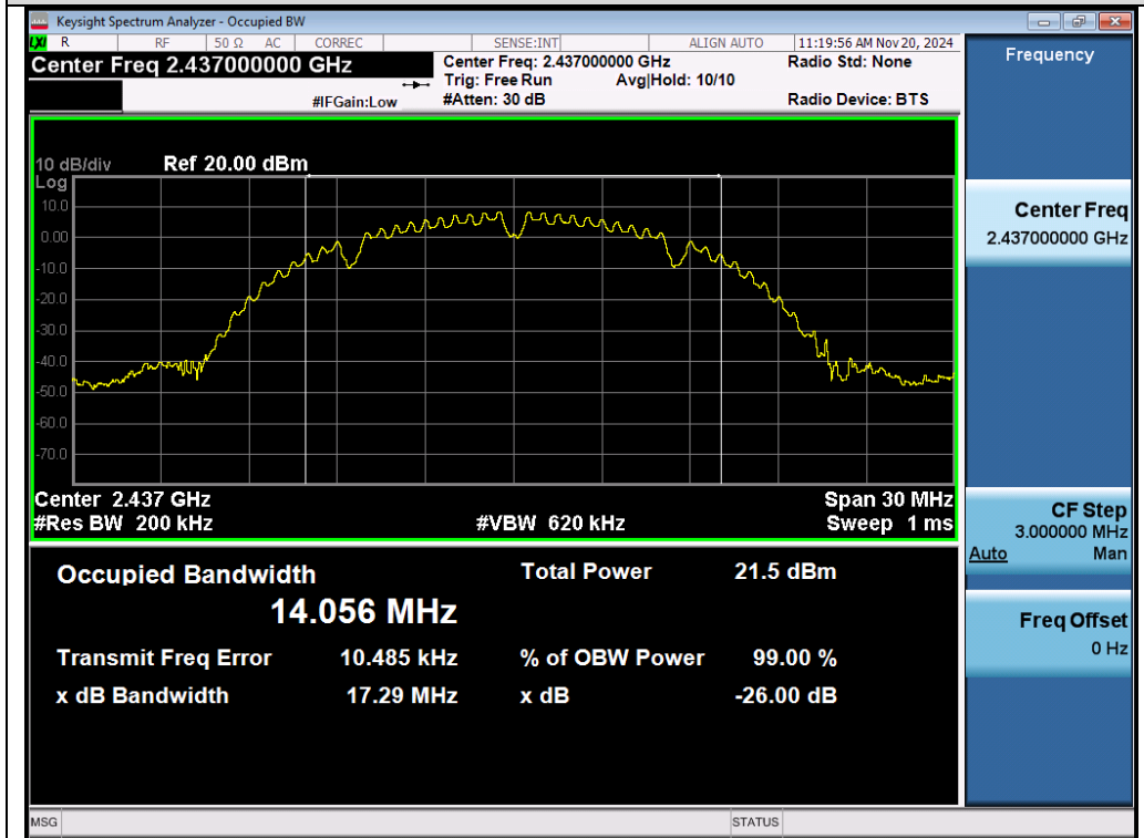
Test_Graph_802.11b_ANT1_2437_1Mbps_OBW
