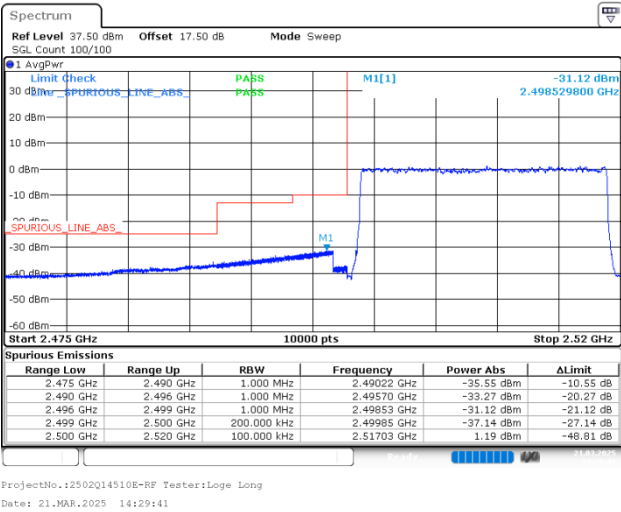
20MHz_Low_16QAM_25@0
