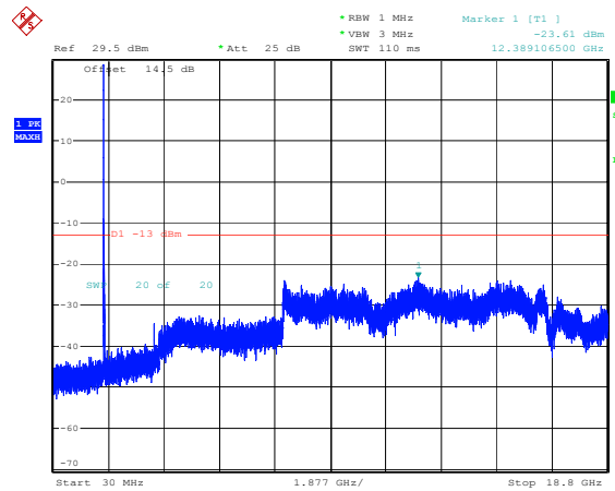
20MHz_Low_QPSK_1@0(30MHz~18.8GHz)
