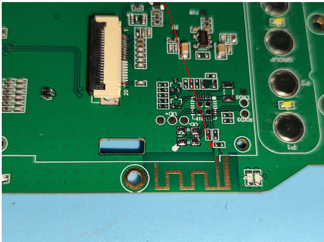
Antenna(Not use)
