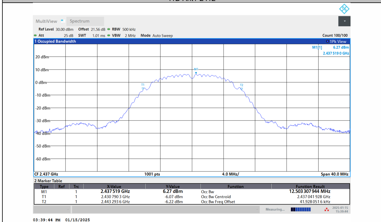
11B-Ant1-2437
