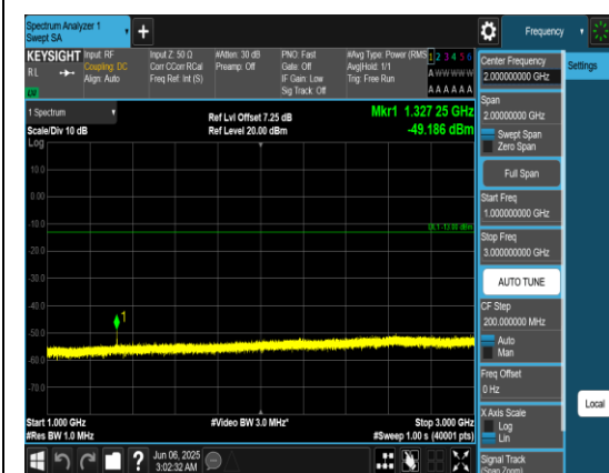
Band71_10MHz_QPSK_133172_1RB#0_1000~3000_1000~3000
