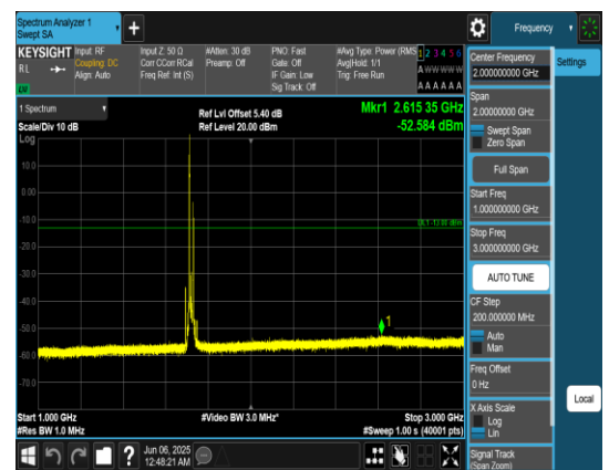
Band66_20MHz_QPSK_132072_1RB#0_1000~3000_000_1000~3000
