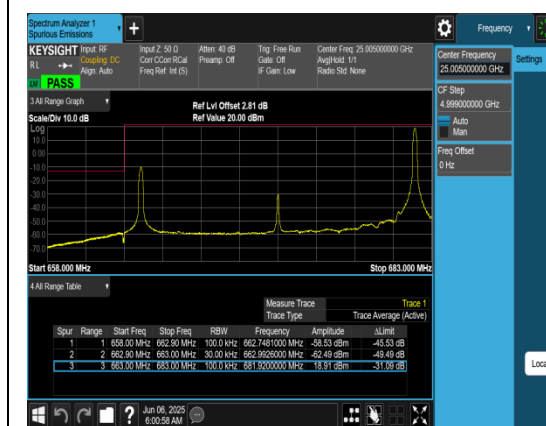
Band71_20MHz_QPSK_133222_1RB#99
