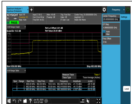
Band71_20MHz_QPSK_133222_100RB#0
