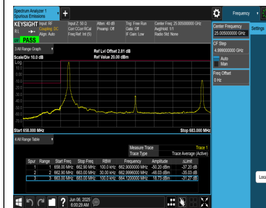
Band71_20MHz_QPSK_133222_1RB#0
