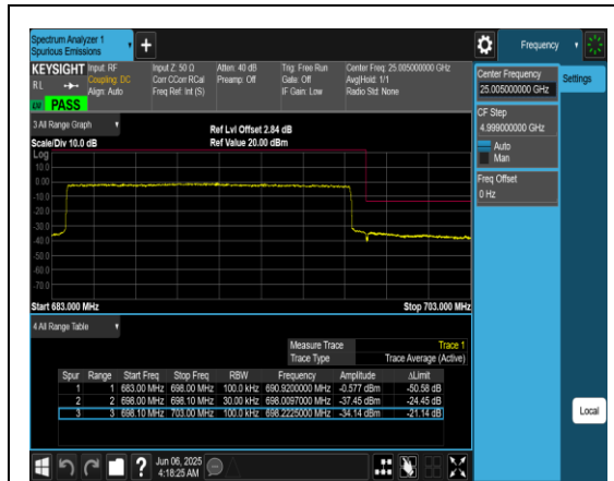
Band71_15MHz_QPSK_133397_75RB#0
