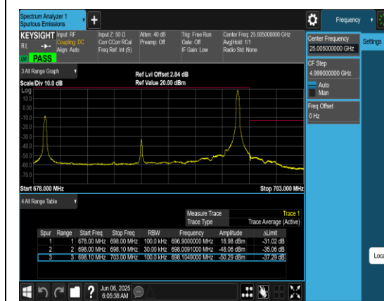
Band71_20MHz_QPSK_133372_1RB#99
