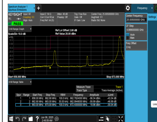
Band71_10MHz_QPSK_133172_1RB#49
