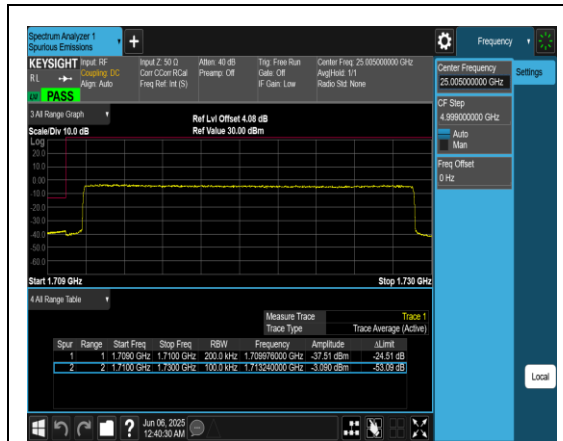
Band66_20MHz_QPSK_132072_100RB#0
