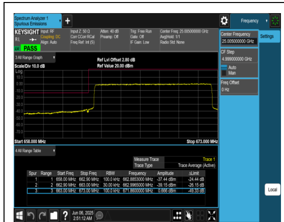
Band71_10MHz_QPSK_133172_50RB#0
