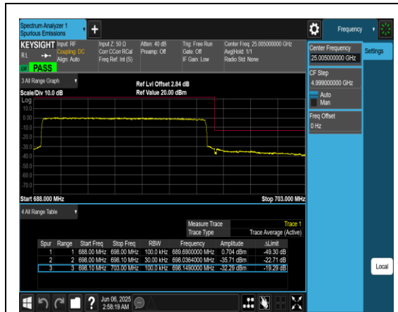
Band71_10MHz_QPSK_133422_50RB#0
