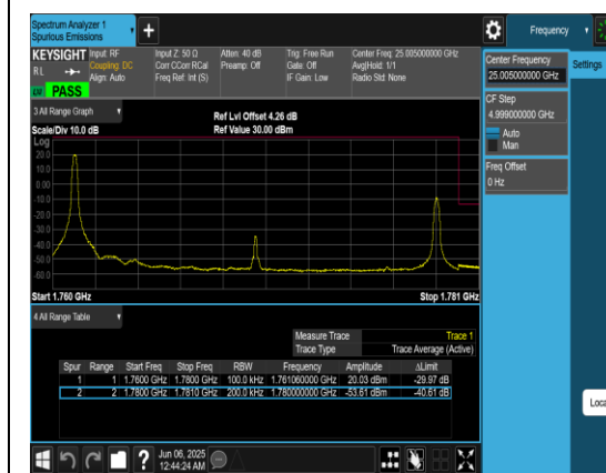
Band66_20MHz_QPSK_132572_1RB#0
