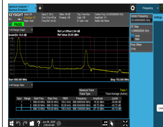
Band71_10MHz_QPSK_133422_1RB#0
