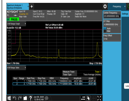
Band66_20MHz_QPSK_132072_1RB#0
