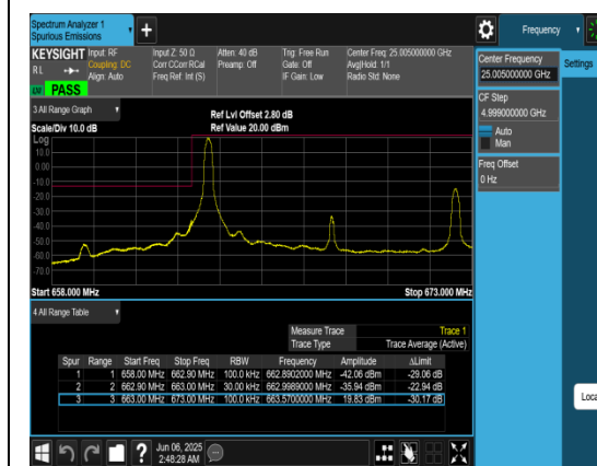
Band71_10MHz_QPSK_133172_1RB#0
