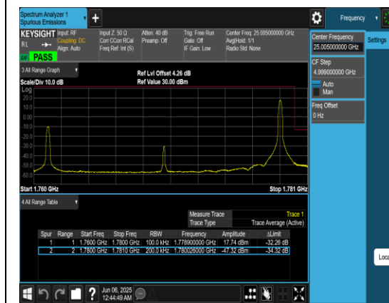
Band66_20MHz_QPSK_132572_1RB#99
