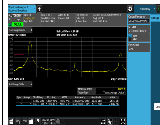
Band2_10MHz_QPSK_18650_1RB#0
