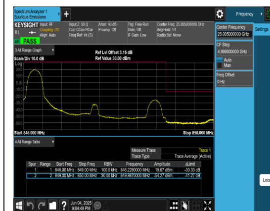
Band5_3MHz_QPSK_20635_1RB#0
