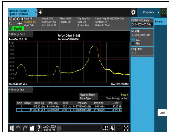
Band5_3MHz_QPSK_20635_1RB#14
