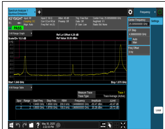
Band2_20MHz_QPSK_18700_1RB#99
