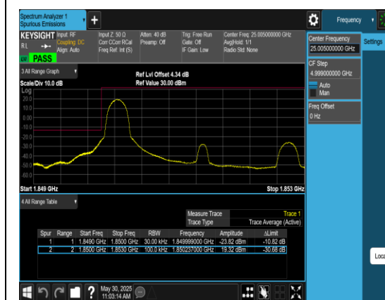
Band2_3MHz_QPSK_18615_1RB#0
