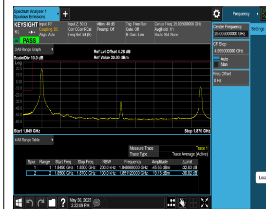
Band2_20MHz_QPSK_18700_1RB#0
