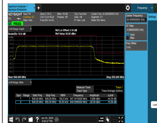
Band5_3MHz_QPSK_20635_15RB#0
