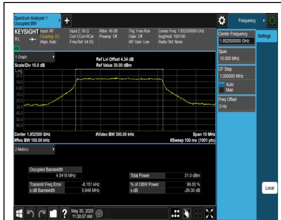
Band2-5MHz-QPSK-18625-25RB#0-PASS
