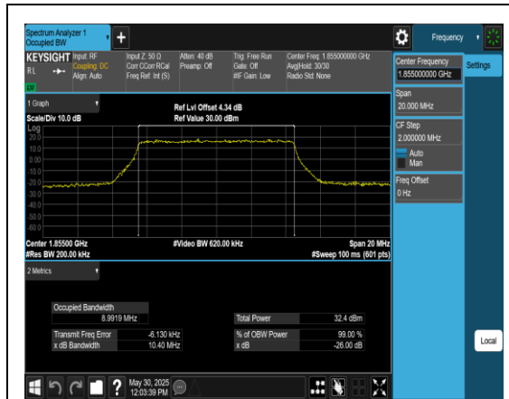
Band2-10MHz-QPSK-18650-50RB#0-PASS
