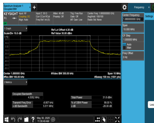
Band2-5MHz-QPSK-18900-25RB#0-PASS
