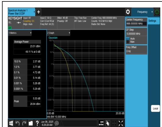
Band71-10MHz-QPSK-133172-1RB#0-PASS
