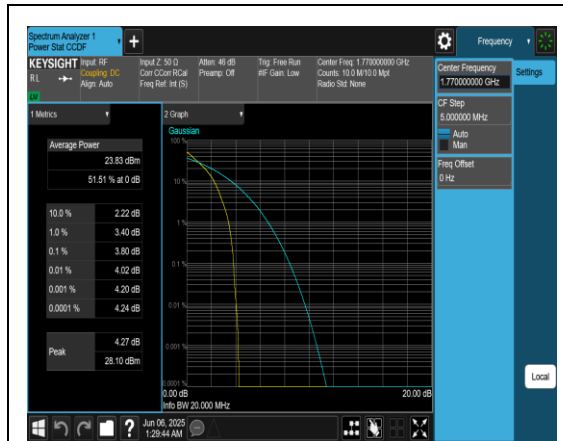
Band66-20MHz-QPSK-132572-1RB#0-PASS
