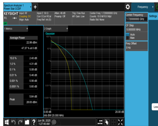
Band66-20MHz-QPSK-132072-1RB#0-PASS
