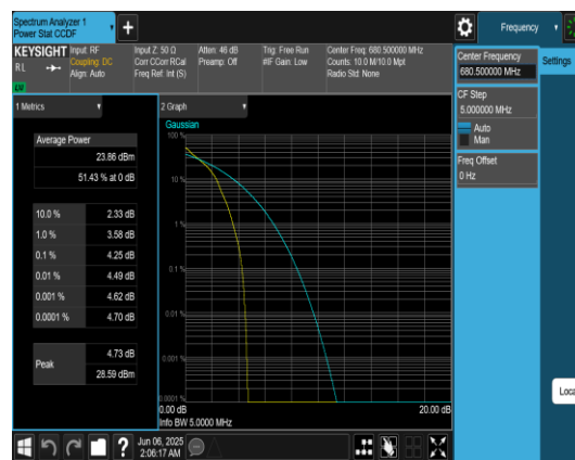
Band71-5MHz-QPSK-133297-1RB#0-PASS
