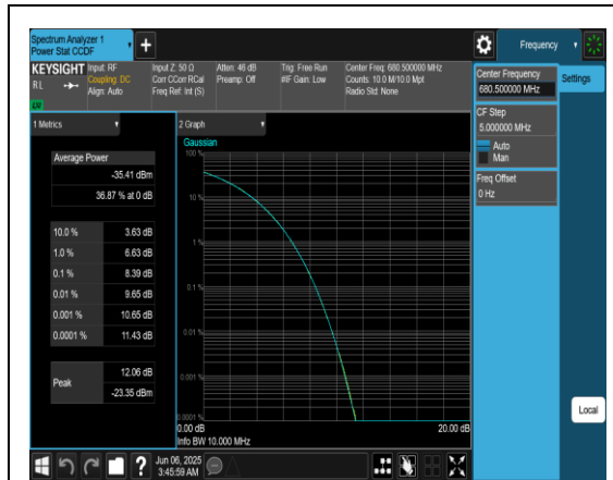
Band71-10MHz-QPSK-133297-1RB#0-PASS
