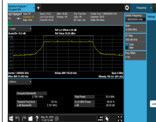
Band2-3MHz-QPSK-18900-15RB#0-PASS
