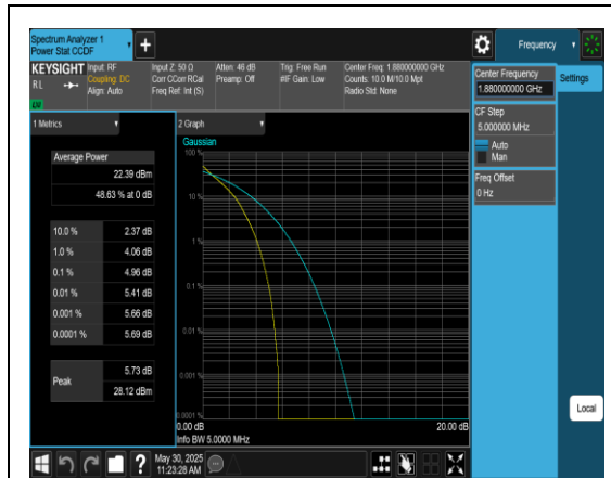
Band2-3MHz-QPSK-18900-15RB#0-PASS
