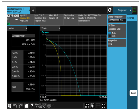
Band2-10MHz-QPSK-18650-1RB#0-PASS
