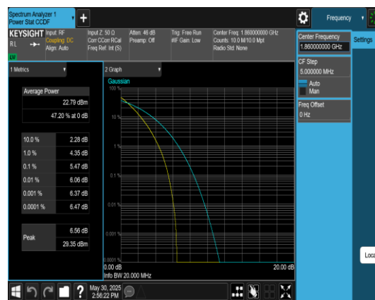
Band2-20MHz-QPSK-18700-100RB#0-PASS
