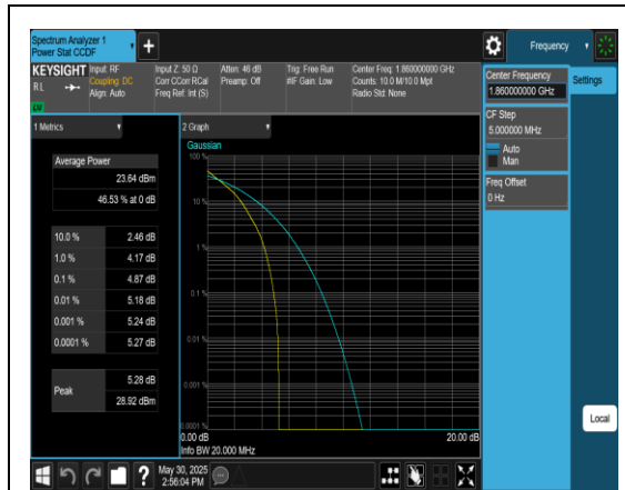
Band2-20MHz-QPSK-18700-1RB#0-PASS
