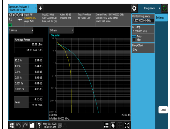
Band2-5MHz-QPSK-19175-1RB#0-PASS
