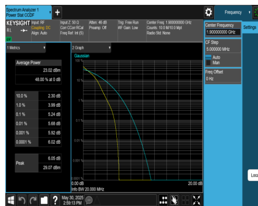
Band2-20MHz-QPSK-19100-1RB#0-PASS
