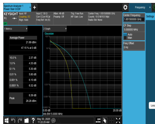
Band2-3MHz-QPSK-18615-15RB#0-PASS
