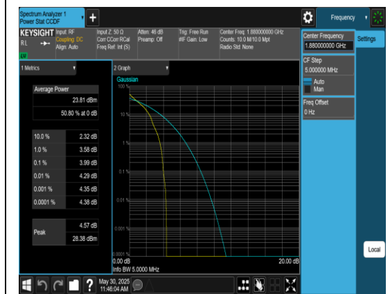
Band2-5MHz-QPSK-18900-1RB#0-PASS
