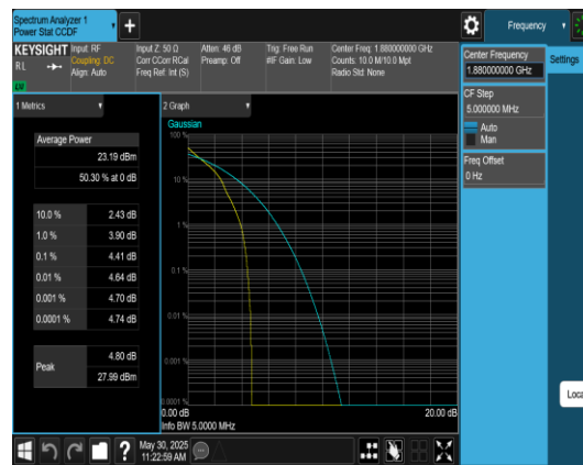
Band2-3MHz-QPSK-18900-1RB#0-PASS
