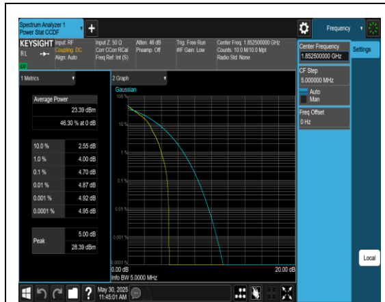
Band2-5MHz-QPSK-18625-1RB#0-PASS
