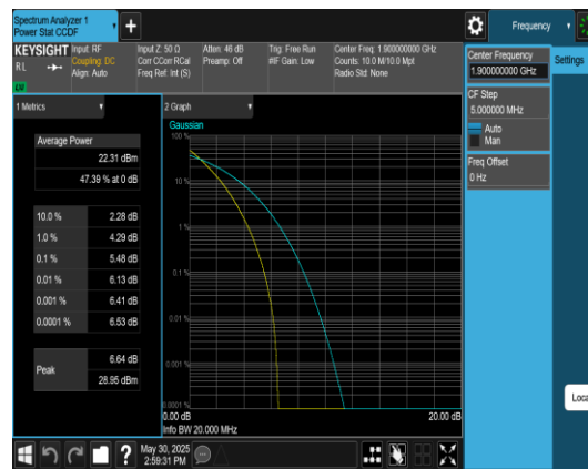
Band2-20MHz-QPSK-19100-100RB#0-PASS
