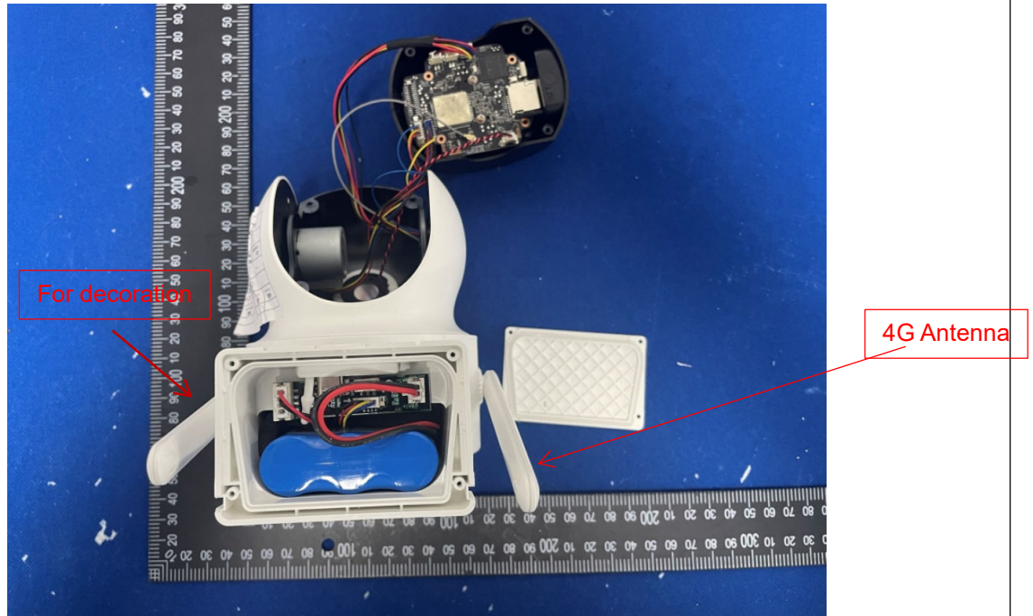
EUT Photo
