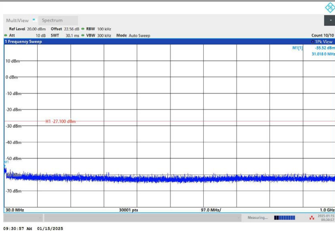
11G-Ant1-2437-30~1000-PASS
