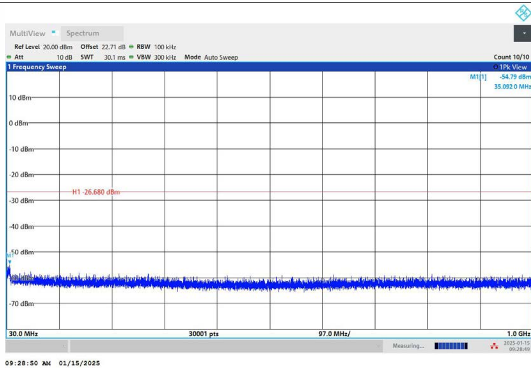
11G-Ant1-2412-30~1000-PASS
