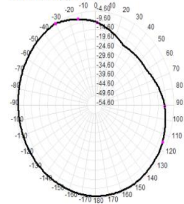
2400.0MHz Total(H), Max=-4.60dBi
