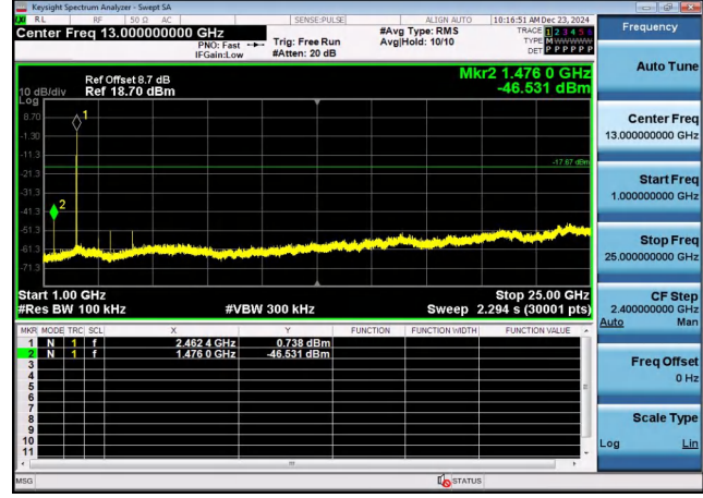
1GHz -25GHz
