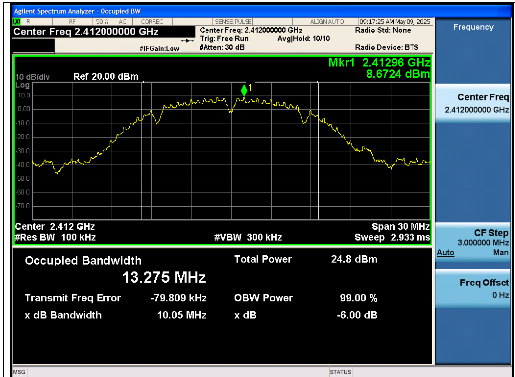
Test_Graph_802.11b_ANT1_2412_1Mbps_DTSPW
