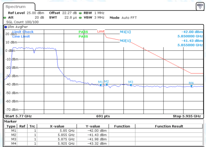
11N40SISO-Ant1-5755-PASS
