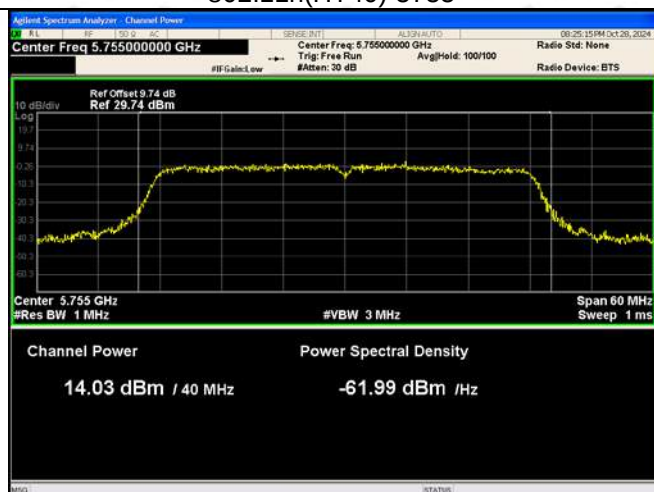
802.11ac(HT80)-5775
