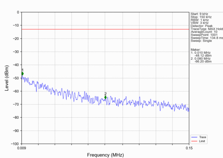
Band66 15MHz QPSK LCH 1717.5MHz RB 1 0 NTNV
