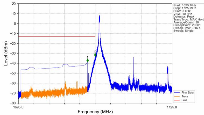
Band66 15MHz QPSK LCH 1717.5MHz RB 1 0 NTNV
