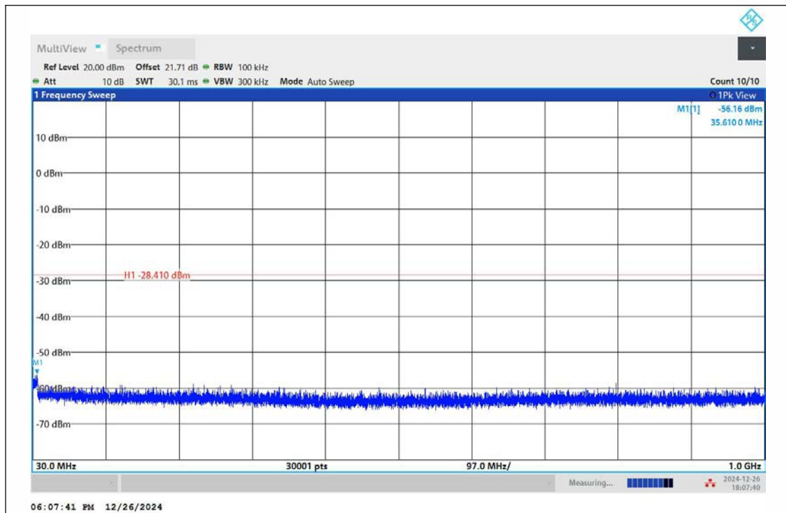
11G-Ant1-2412-30~1000-PASS
