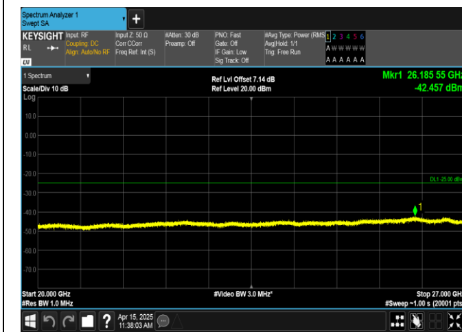
Band41-20MHz-QPSK-41490-1RB#0-20000~27000-PASS
