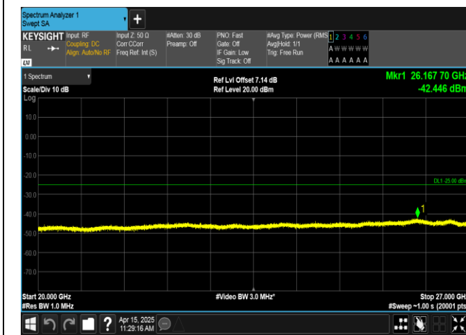
Band41-20MHz-QPSK-39750-1RB#0-20000~27000-PASS
