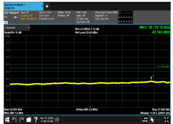
Band41-20MHz-QPSK-41490-1RB#99-20000~27000-PASS
