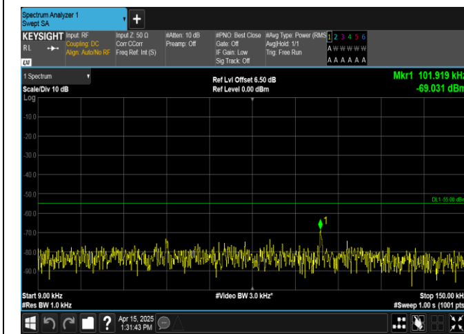
Band41-10MHz-QPSK-41540-50RB#0-0.009~0.15-PASS
