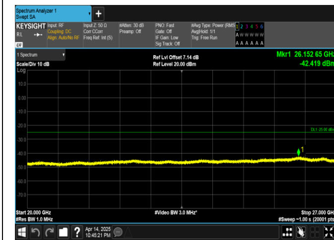
Band41-5MHz-QPSK-41565-1RB#0-20000~27000-PASS
