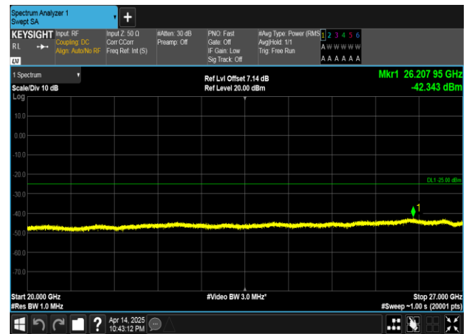
Band41-5MHz-QPSK-40620-25RB#0-20000~27000-PASS
