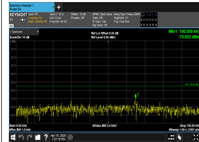
Band41-10MHz-QPSK-39700-50RB#0-0.009~0.15-PASS
