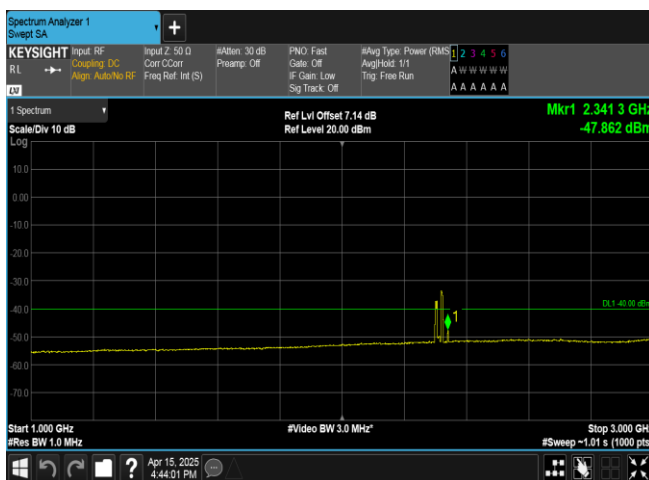
Band40(2305-2315)-10MHz-QPSK-38750-1RB#49-1000~3000-PASS
