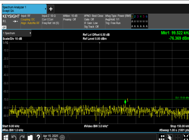
Band40(2305-2315)-10MHz-QPSK-38750-50RB#0-0.009~0.15-PASS
