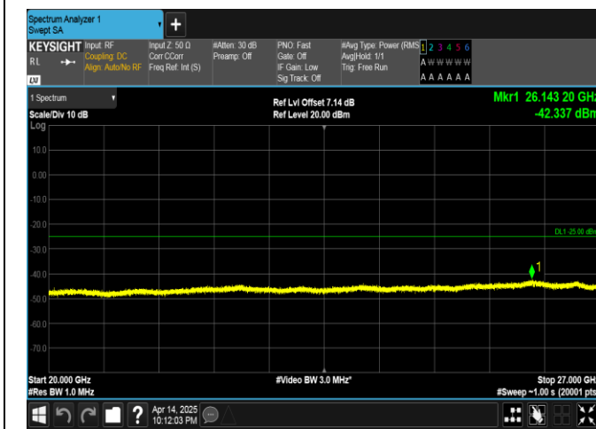
Band38-20MHz-QPSK-38150-1RB#0-20000~27000-PASS
