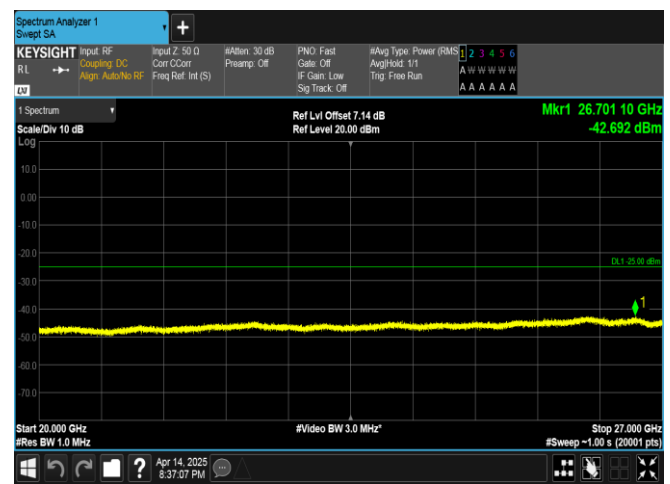
Band38-5MHz-QPSK-38000-25RB#0-20000~27000-PASS
