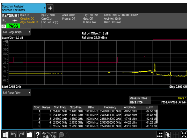
Band38-20MHz-QPSK-37850-1RB#0-PASS
