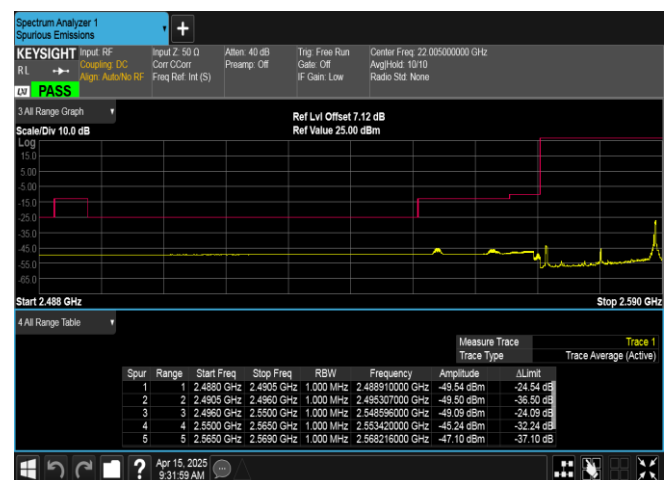
Band38-20MHz-QPSK-37850-1RB#99-PASS
