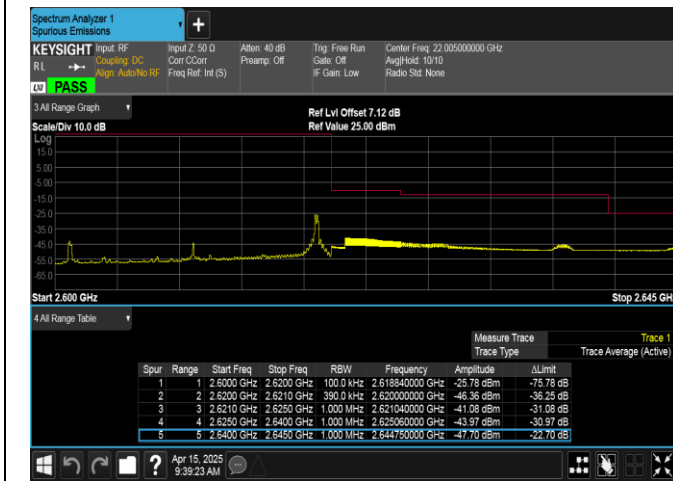
Band38-20MHz-QPSK-38150-1RB#99-PASS
